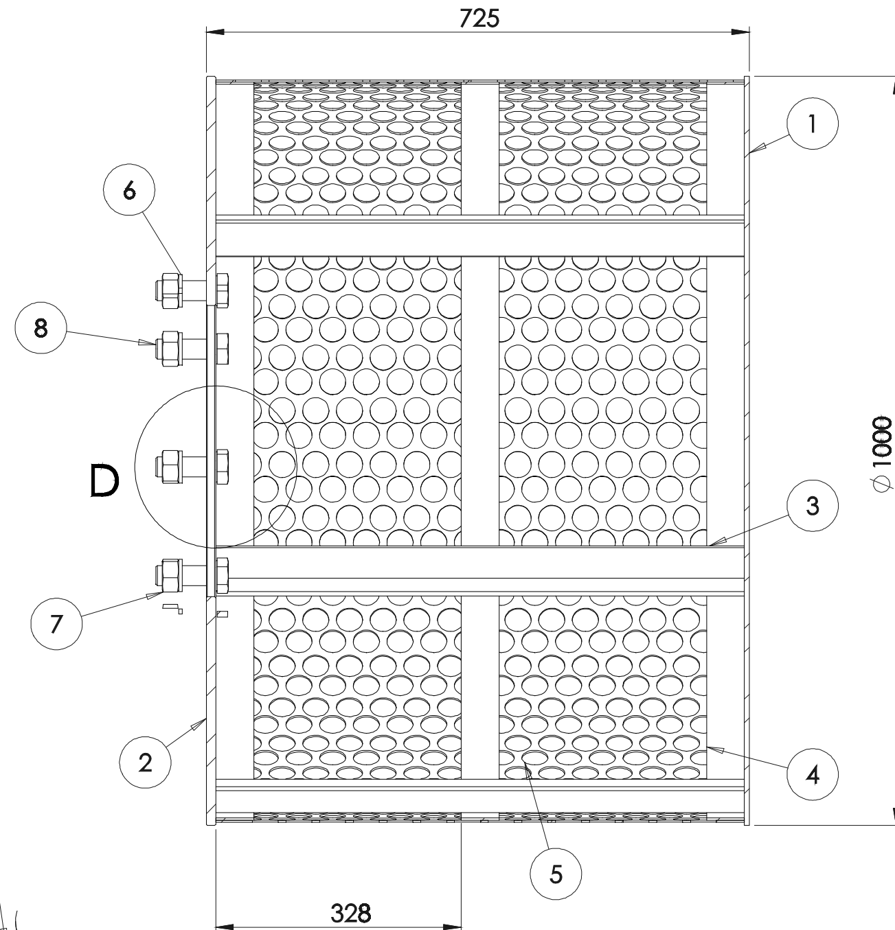
SEÇÃO A-A ESCALA 1 : 7
