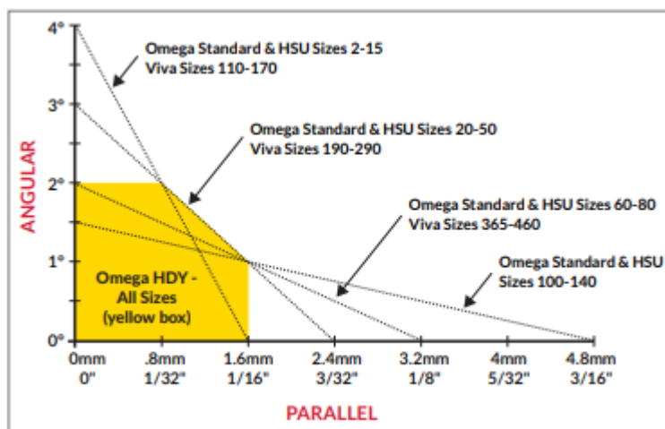
Gráfico 1 – Tolerância angular e linear para cada tamanho de acoplamento
