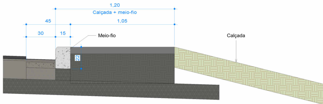
4 DETALHE MEIO-FIO 1 : 10
