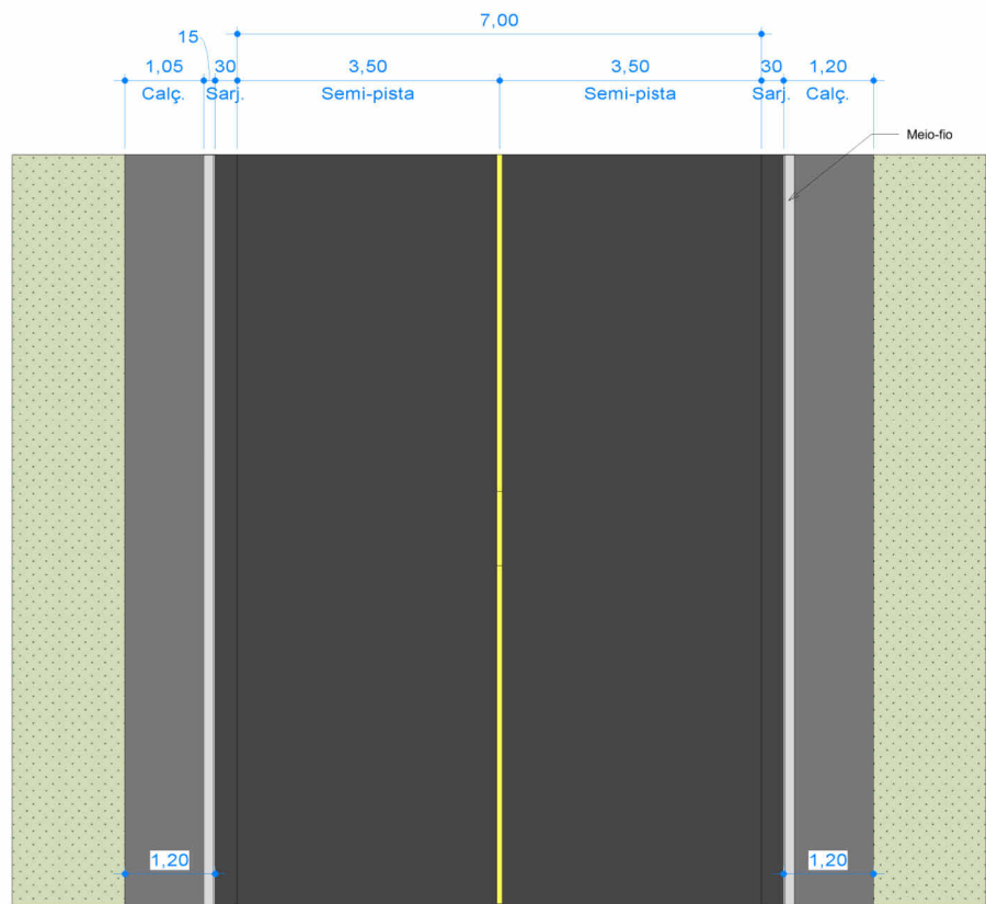
1 PLANTA BAIXA 1 : 50
