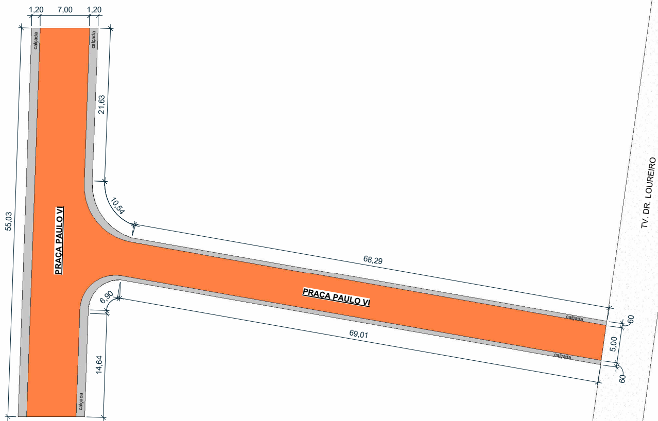
4 DETALHE DA RUA 1:200
