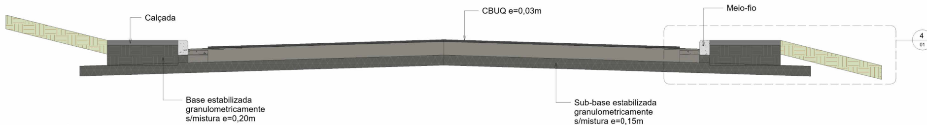
3 SEÇÃO DA PISTA 1 : 25
