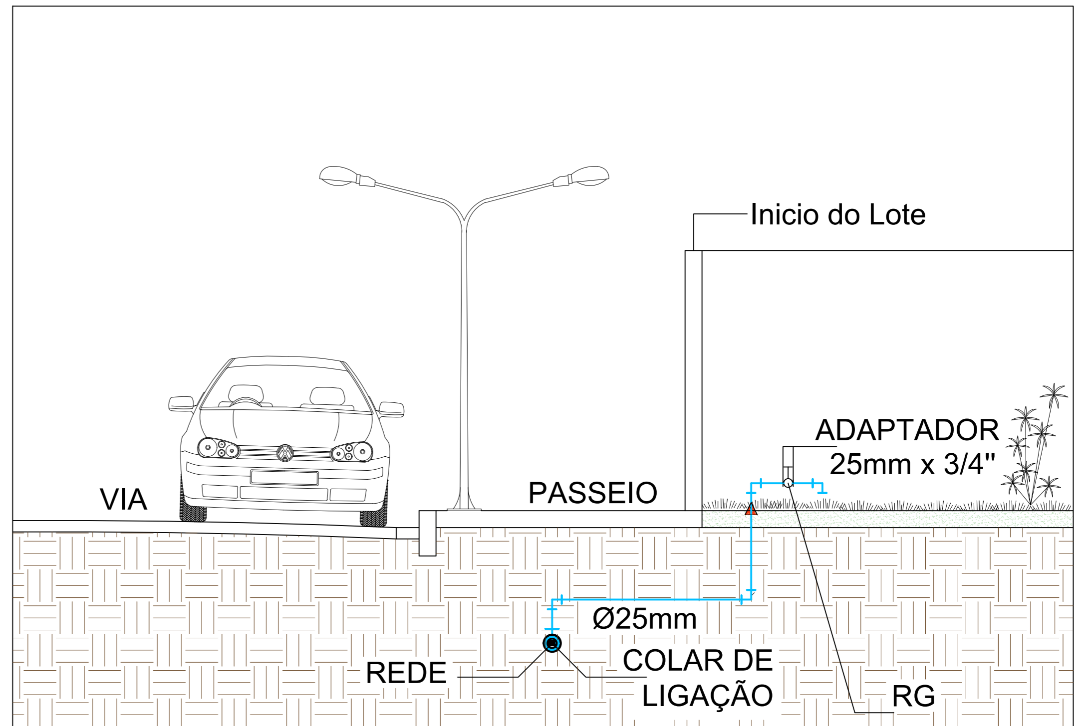
DETALHE DE ENTRADA DE ÁGUA - CAVALETE LIGAÇÃO DOMICILIAR ESC: SEM ESCALA
