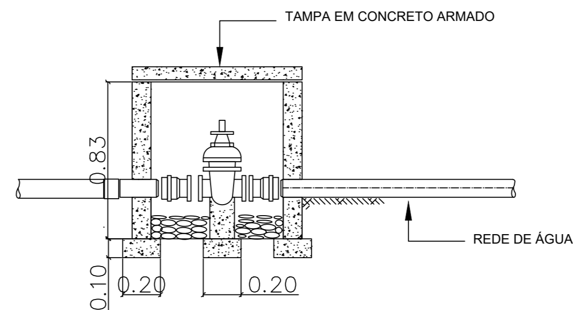
DET. DA CAIXA DE REGISTRO DE MANOBRA
