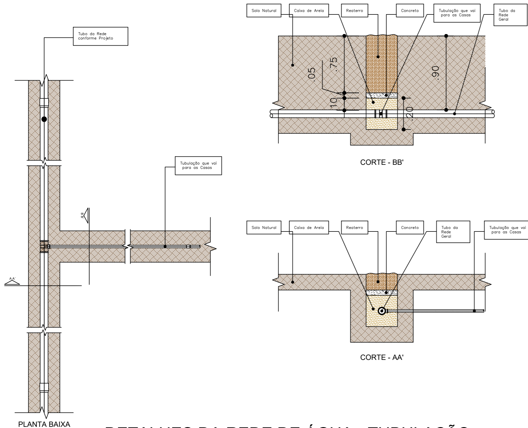
DETALHES DA REDE DE ÁGUA - TUBULAÇÃO ESC: SEM ESCALA
