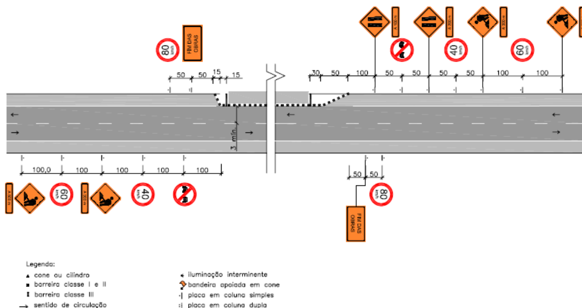
Figura 15 - Croqui de sinalização
