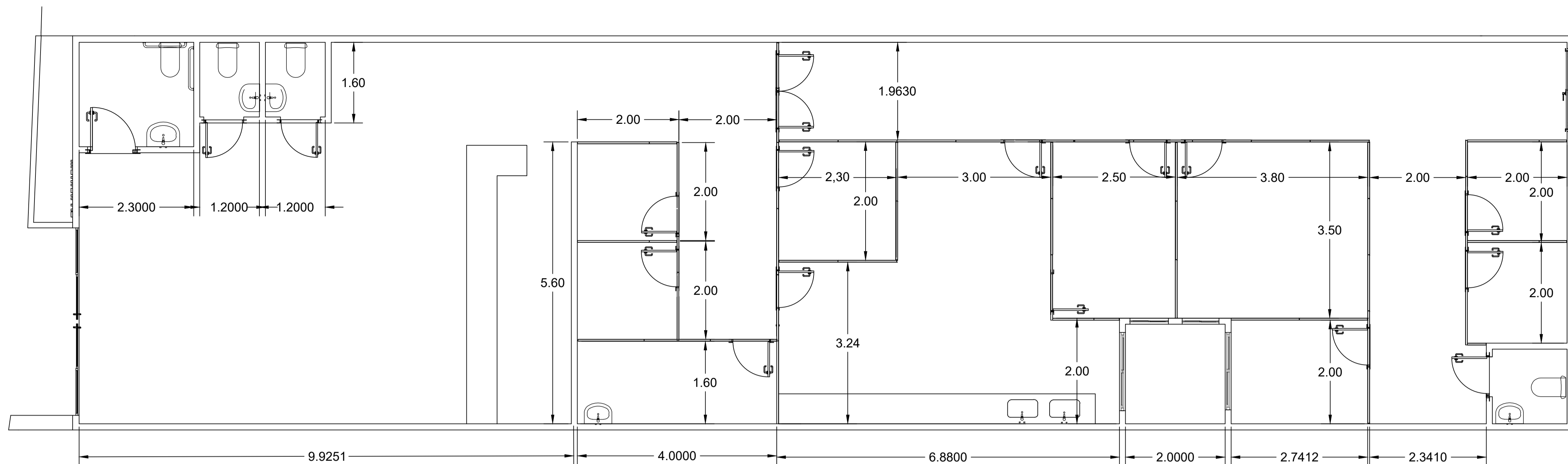
2 PLANTA DE DRY WALL 1:100
