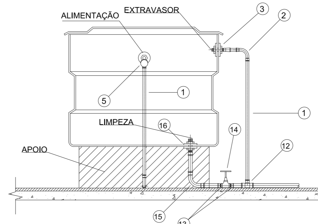
INSTALAÇÃO DE CAIXA D'ÁGUA ESCALA 1:10
