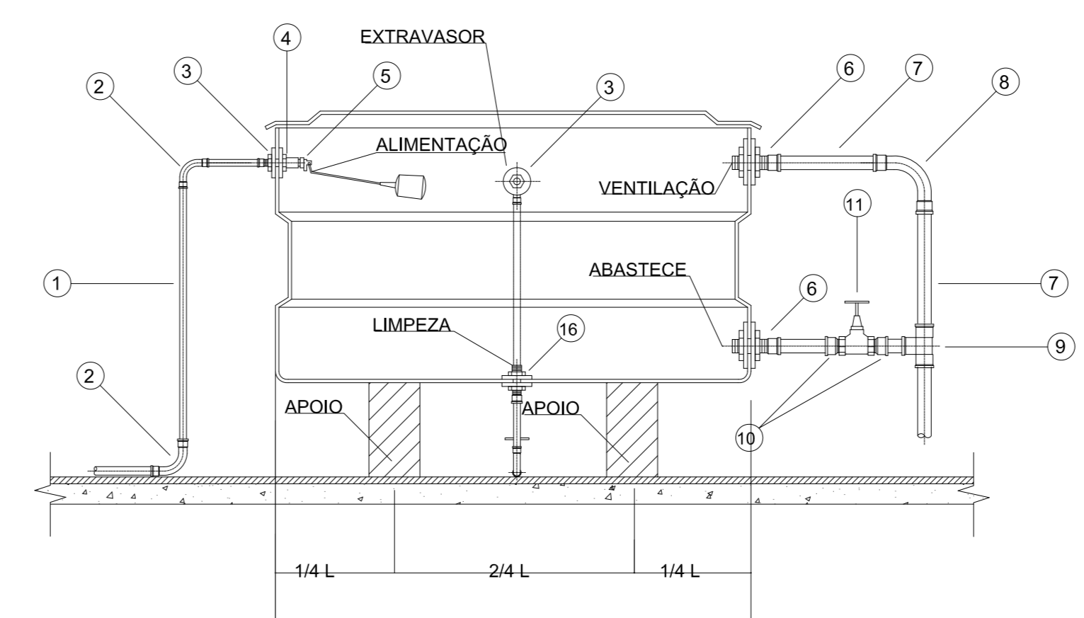
CORTE LONGITUDINAL ESCALA 1:10
