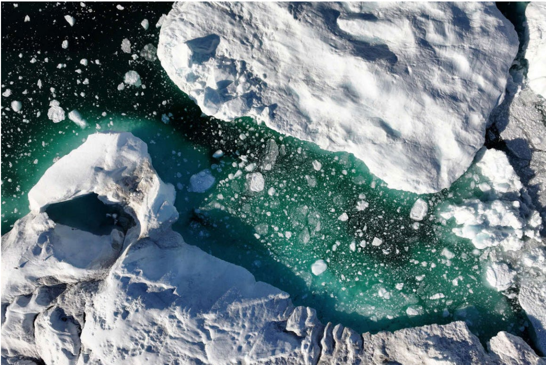
A pesquisa, publicada recentemente, indica que a Groenlândia já perdeu completamente sua calota polar em um período interglacial passado
