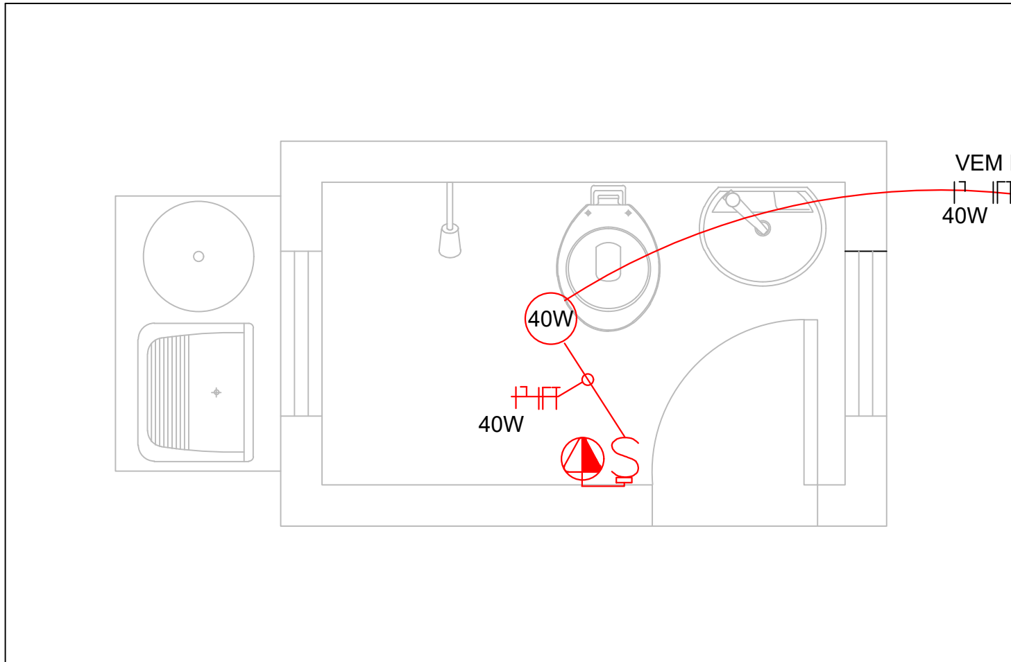
PLANTA BAIXA - ELÉTRICO ESC.: 1:20
