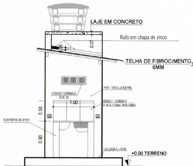
VISTA LAT. _BANHEIRO ESC.: 1:50
