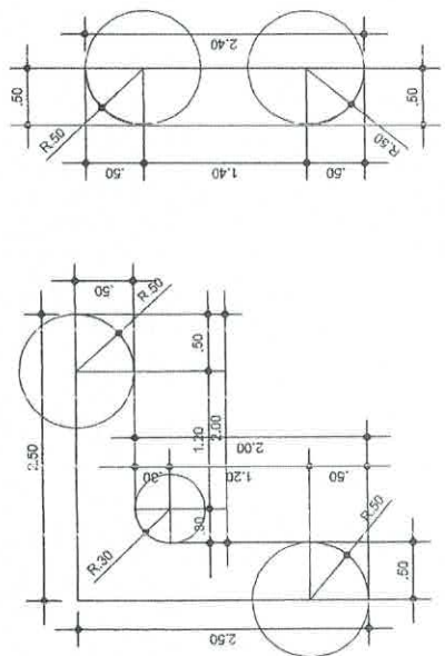
DETALHE 02 - CANTEIROS ESC. 1:25
