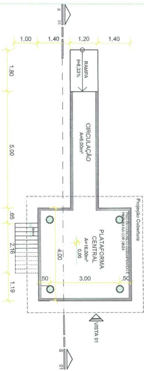
PLANTA BAIXA - PLATAFORMA PRINCIPAL ESC 1/100
