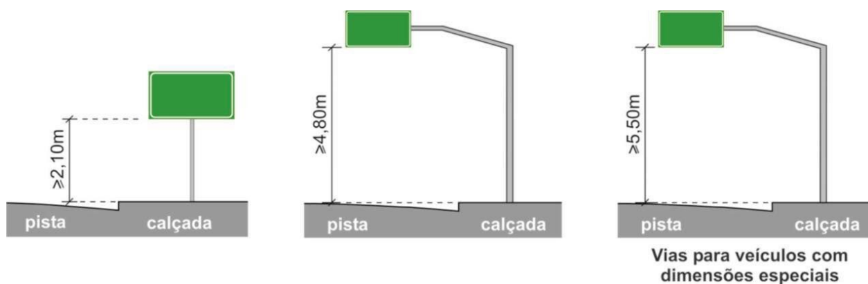
Figura 3 - Vista frontal
