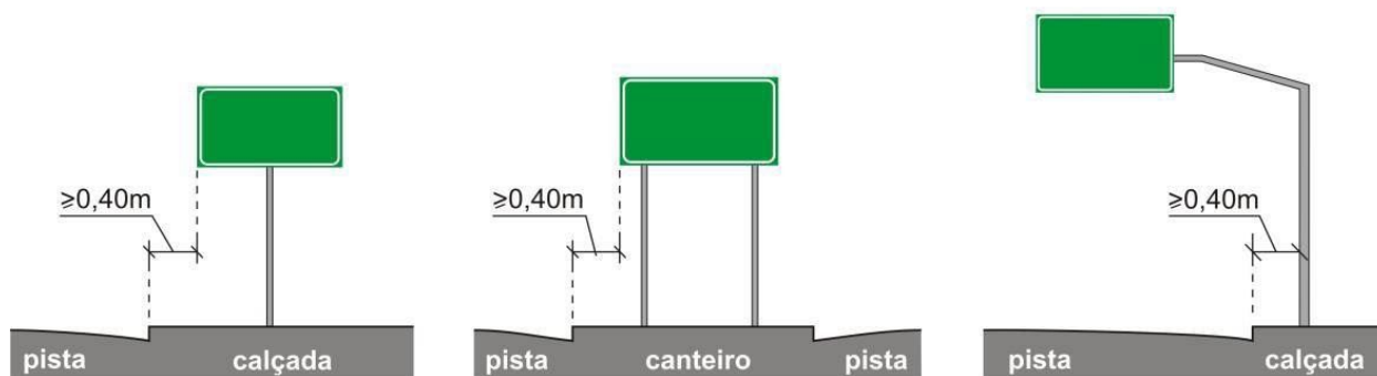
Figura 4 - Vista frontal (afastamento)
