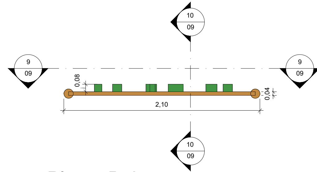
8 Planta Baixa 1 : 25
