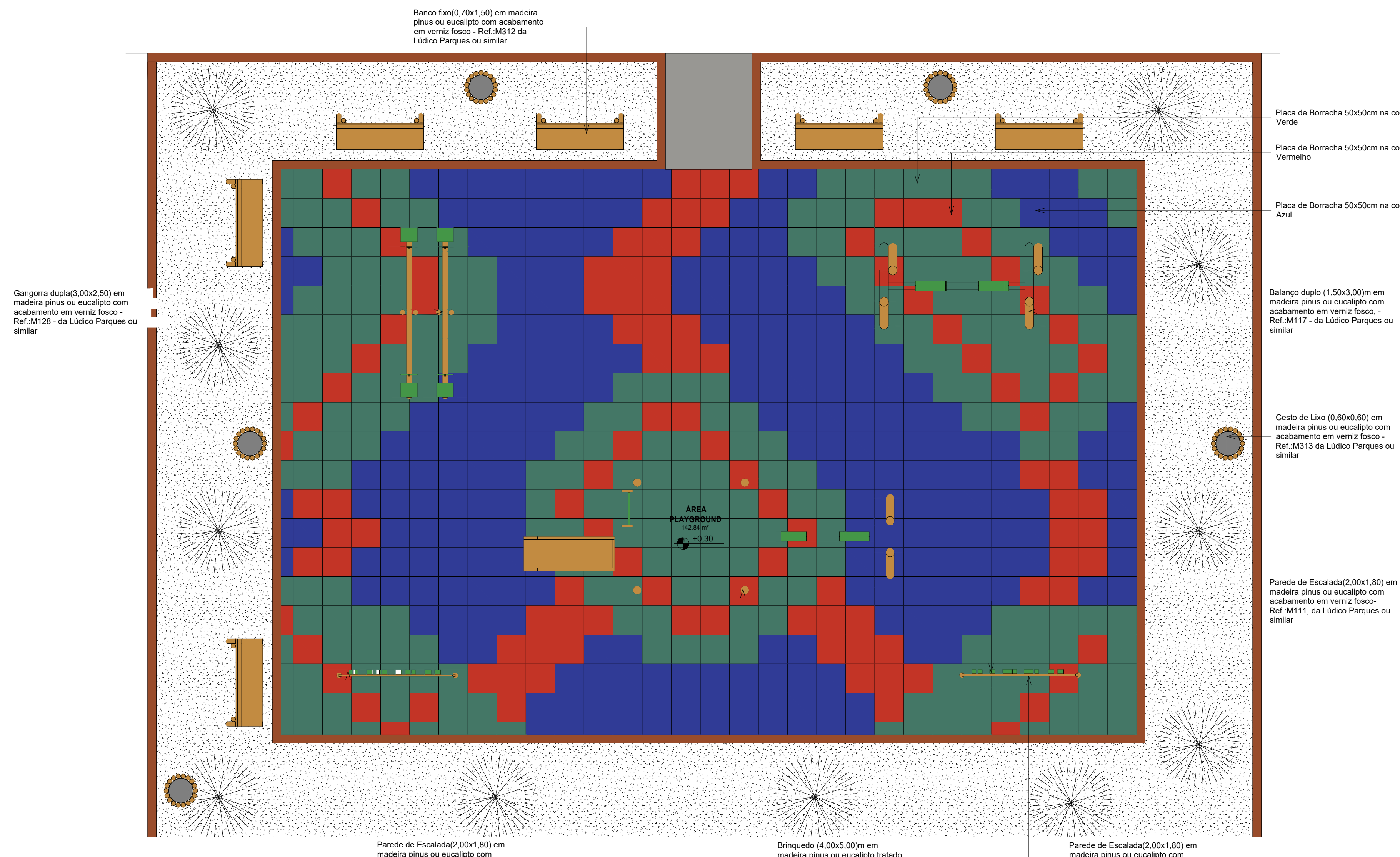
1 Planta Baixa - Playground Layout 1 : 50
