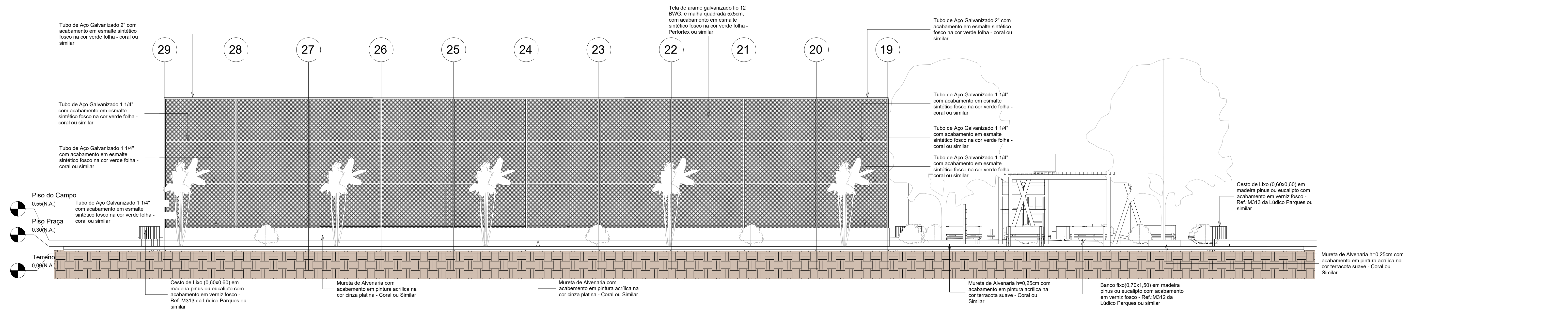
1 Fachada Leste 1 : 75
