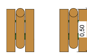
13 Corte 13 1 : 25
