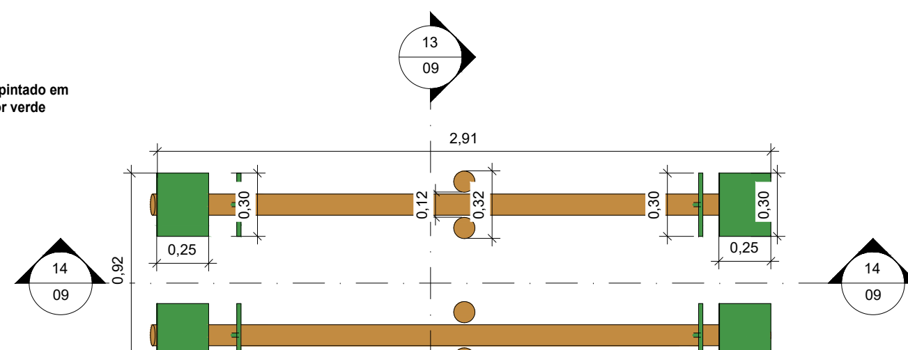
12 Planta Baixa 1 : 25
