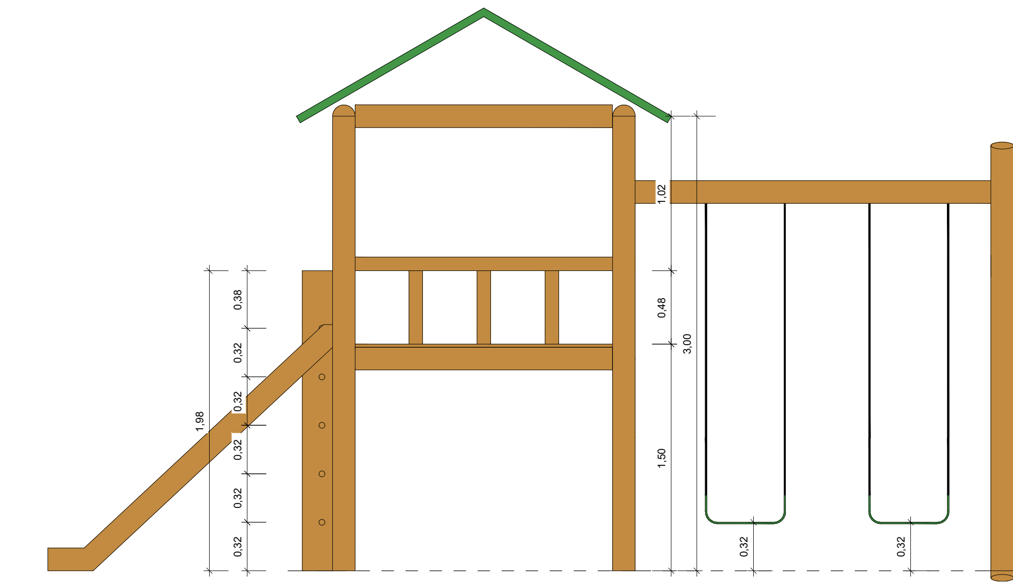
2 Vista 2 1 : 25
