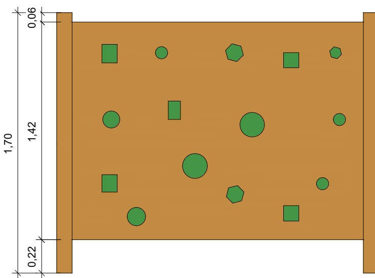
9 Vista 9 1 : 25
