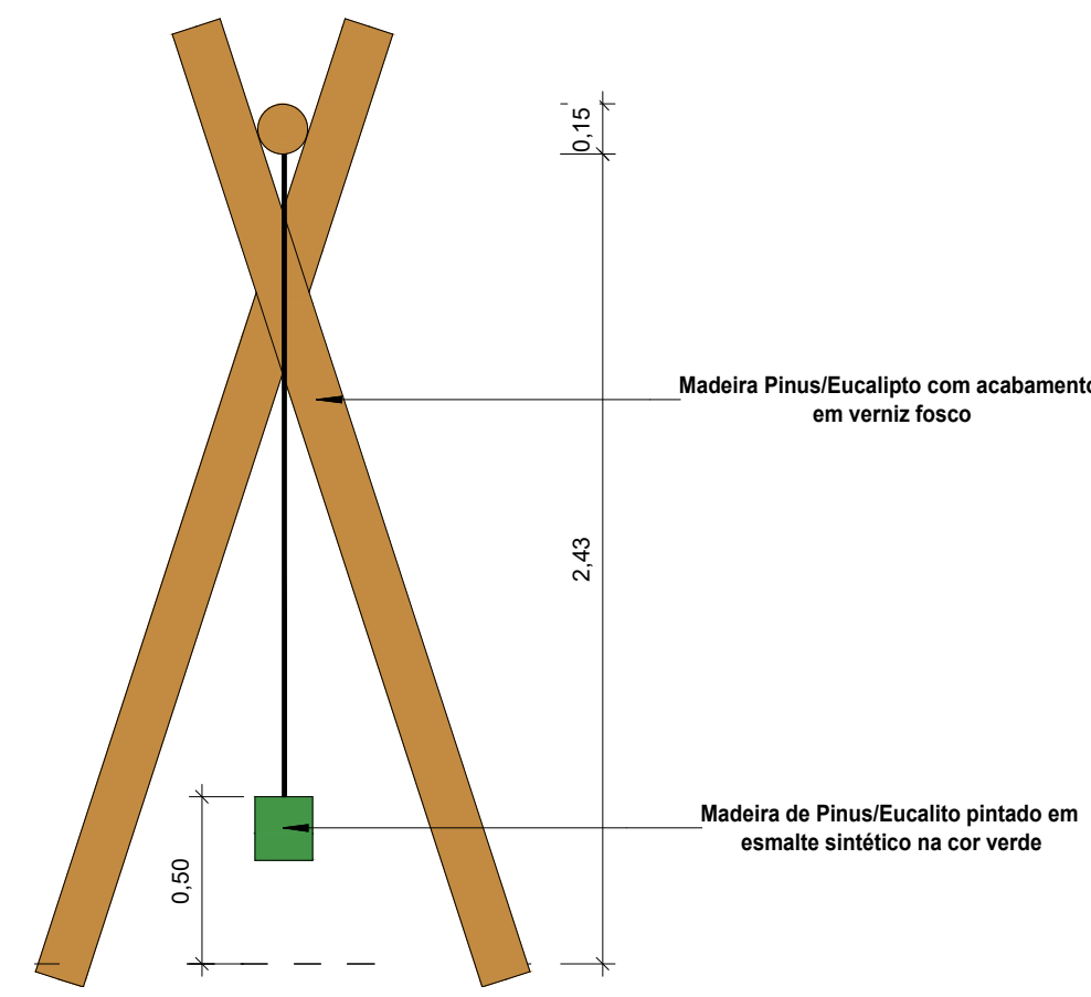
5 Corte 5 1 : 25
