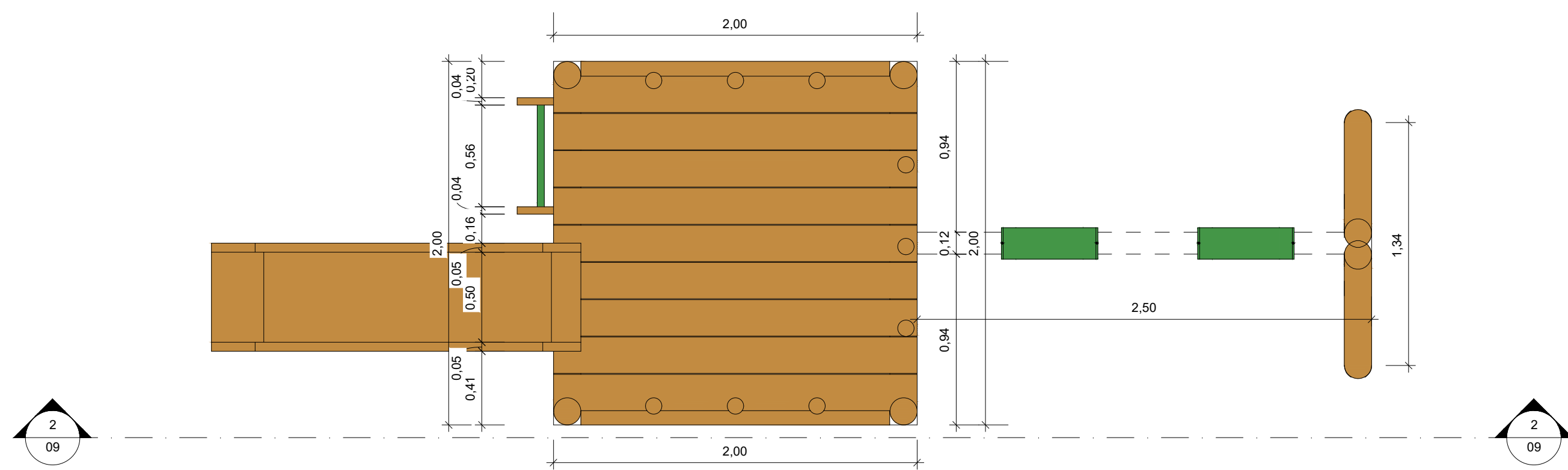
3 Planta Baixa 1 : 25
