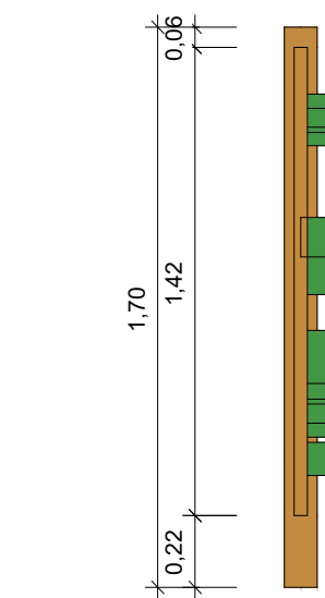
10 Corte 10 1 : 25
