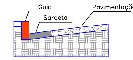
DETALHAMENTO SARGETA 1:75
