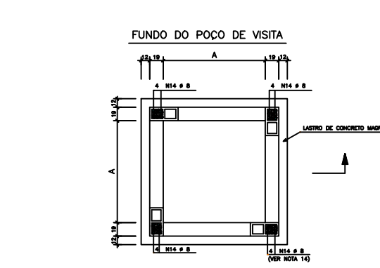
DETALHAMENTO PV 1:75
