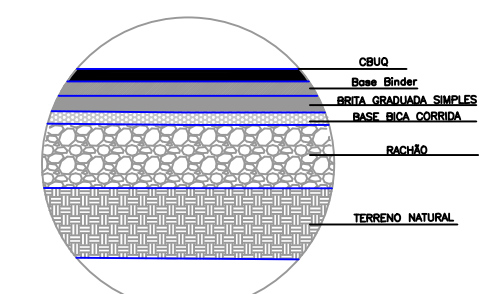
DETALHAMENTO CAMADAS DA PAV SEM ESCALA
