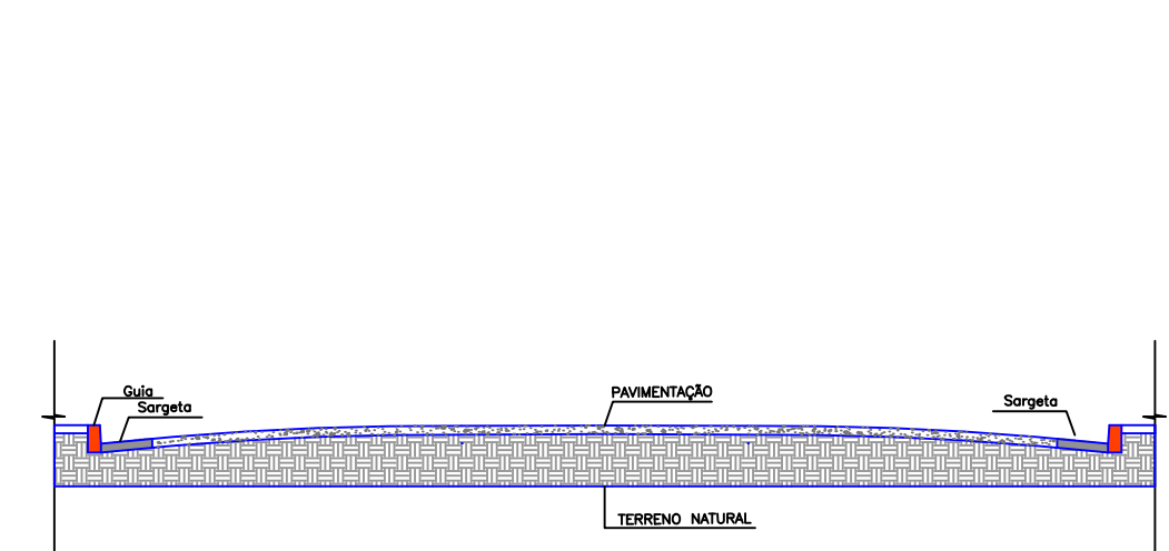
DETALHAMENTO RUA 1:50
