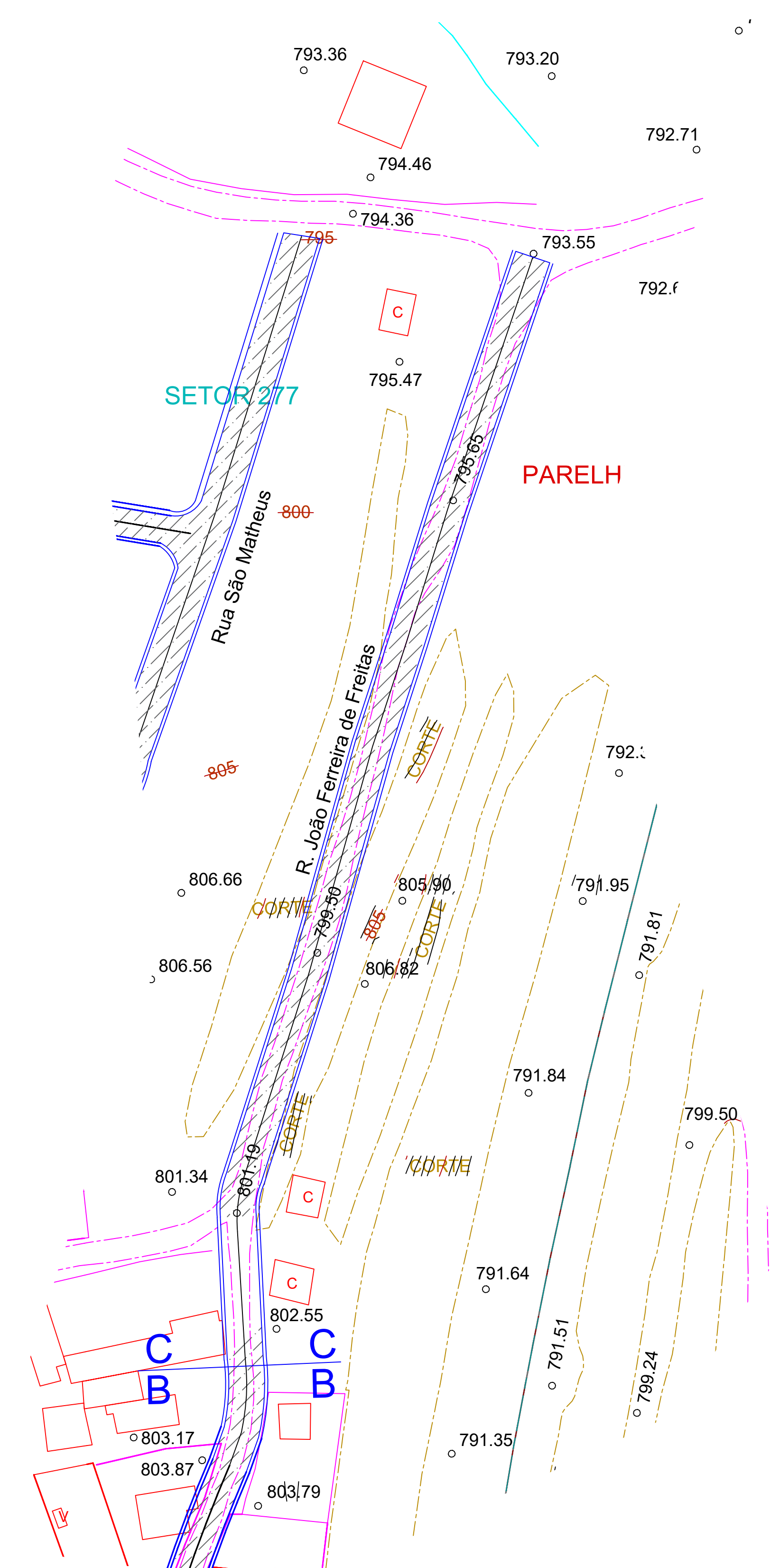
RUA PAULO DE FREITAS TRECHO C 1:500
