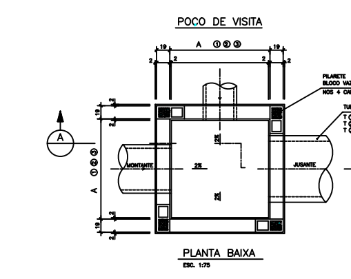
DETALHAMENTO PV 1:75
