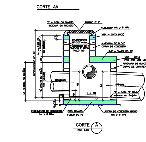
DETALHAMENTO PV 1:75
