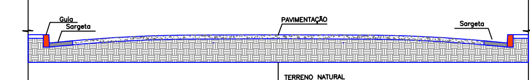
DETALHAMENTO RUA 1:50
