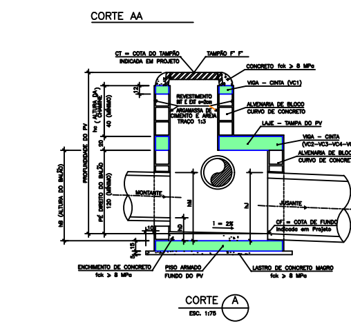
DETALHAMENTO PV 1:75
