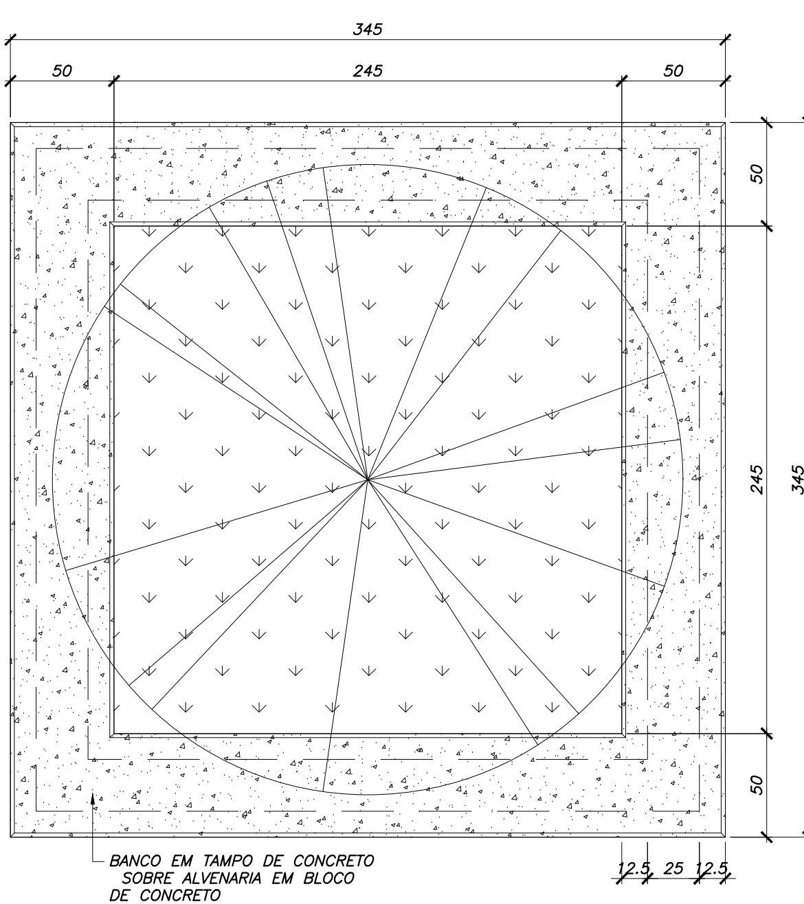
DETALHE - BANCO PRAÇA ESC. 1:25
