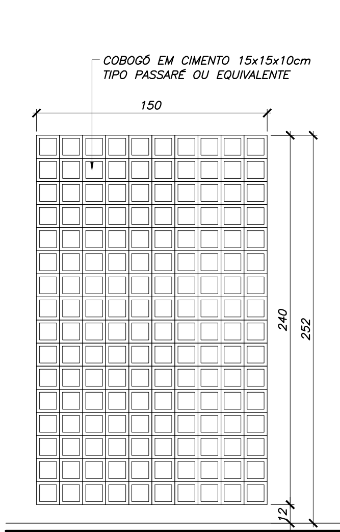
ELEMENTO VAZADO EV-01
