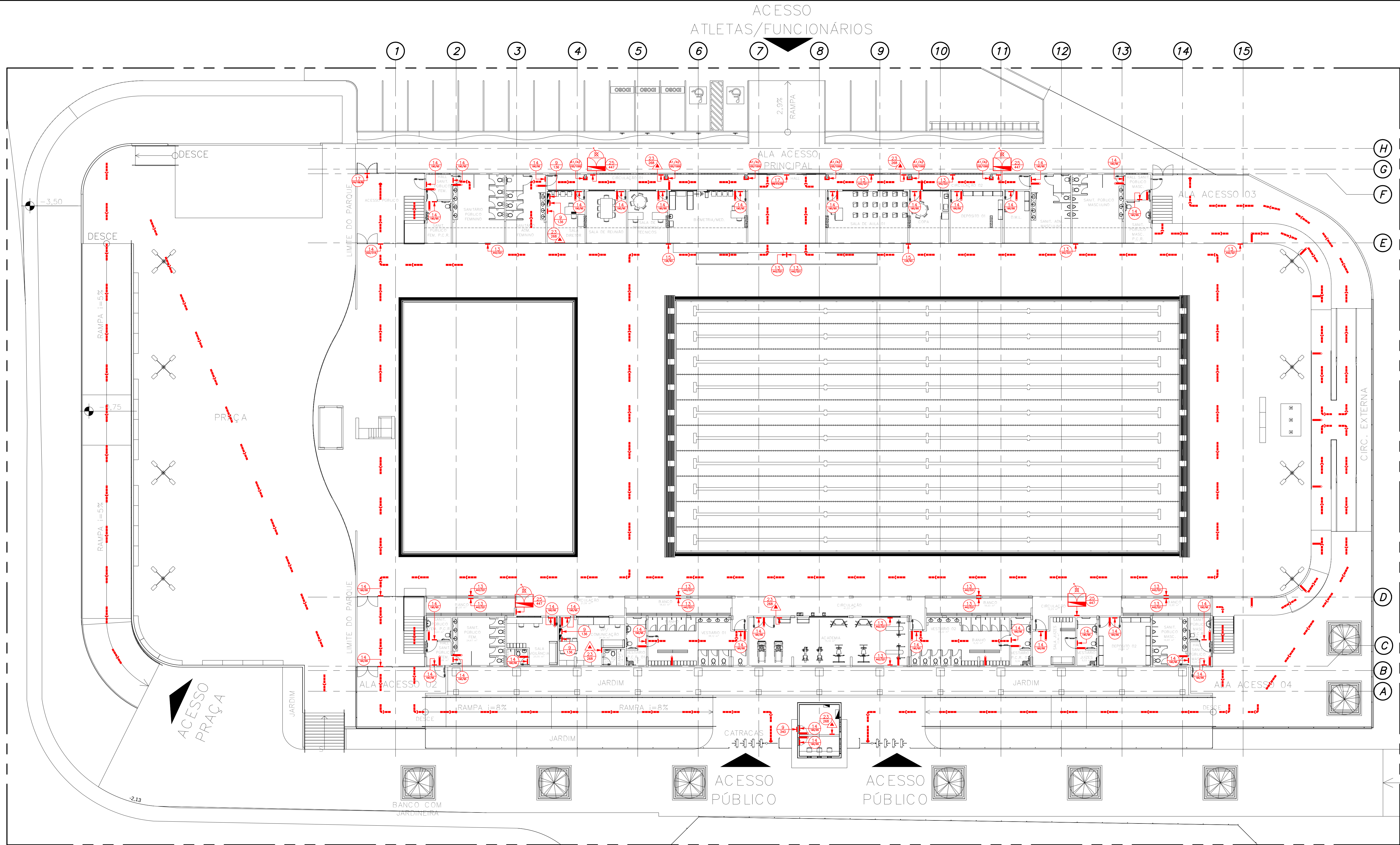
ROTA DE FUGA, ILUMINAÇÃO, SINALIZAÇÃO E EXTINTORES ESC. 1:175
