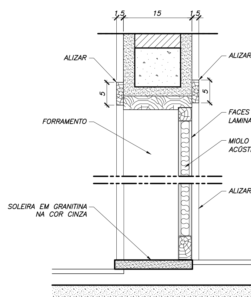
DET. LATERAL PORTAS DE MADEIRA
