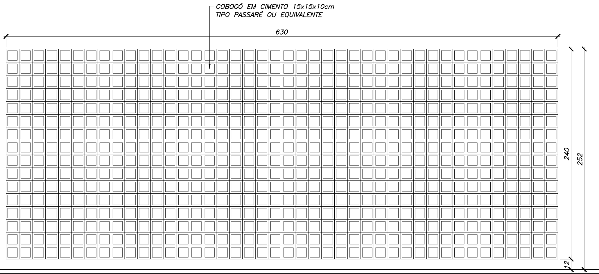
ELEMENTO VAZADO EV-03
