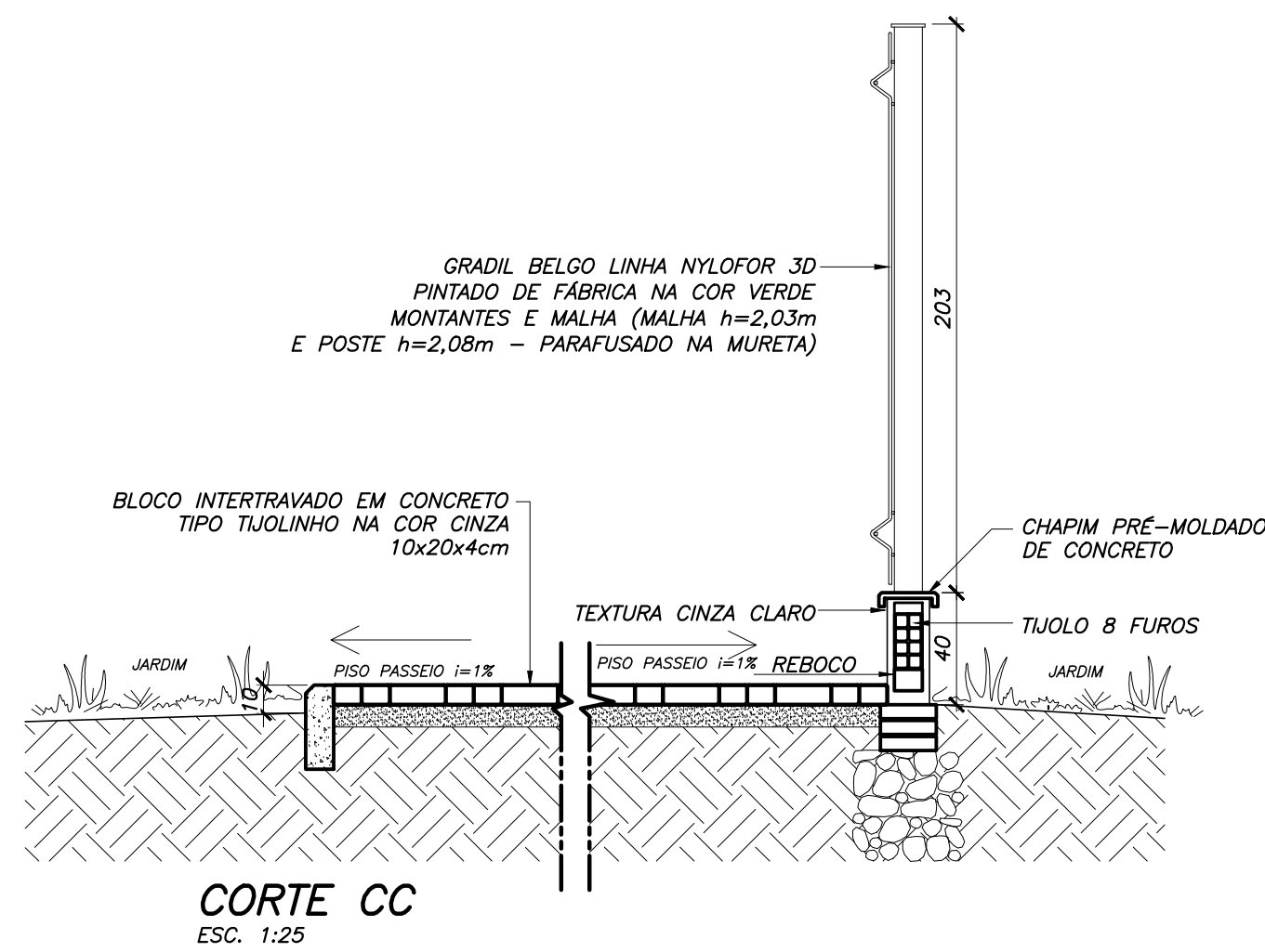
DETALHE DE PASSEIO E GRADIL PERIMETRAL ESC. 1:25
