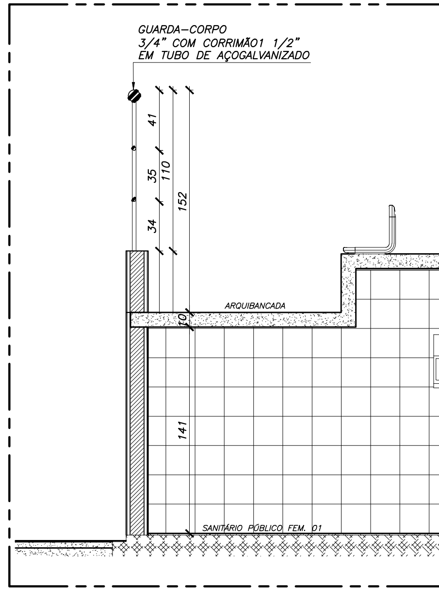
DETALHE - GUARDA-CORPO - ARQUIBANCADA ESC. 1:25
