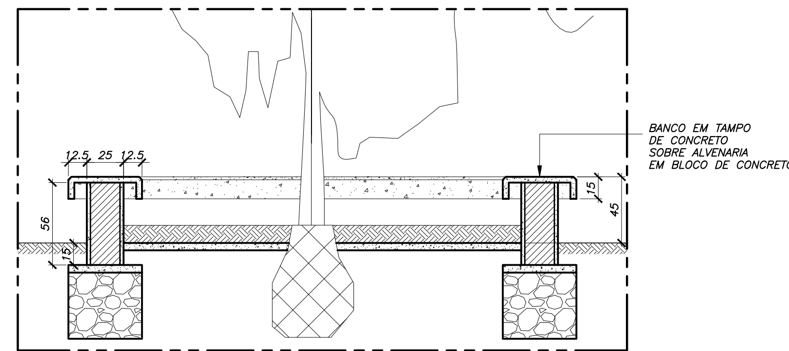
CORTE DD ESC. 1:25
