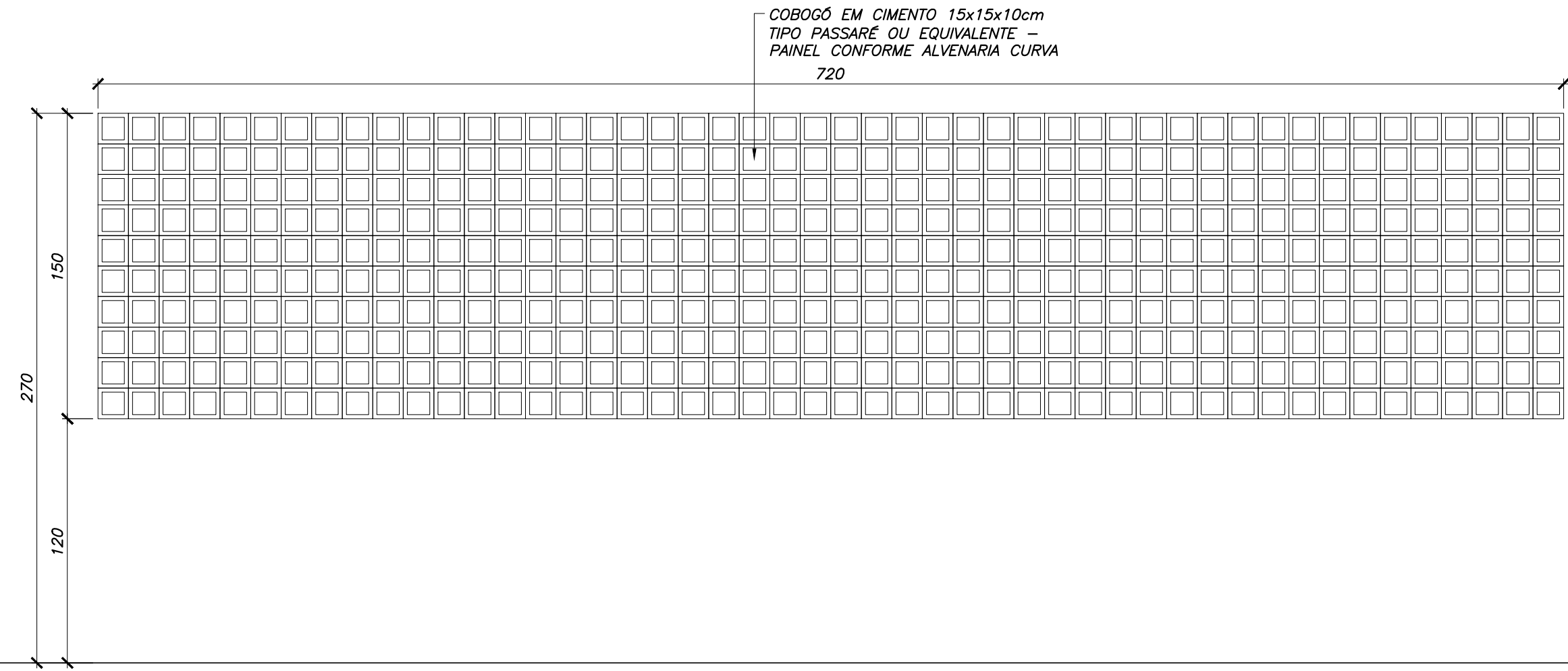
ELEMENTO VAZADO EV-07
