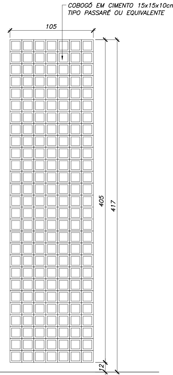
ELEMENTO VAZADO EV-04
