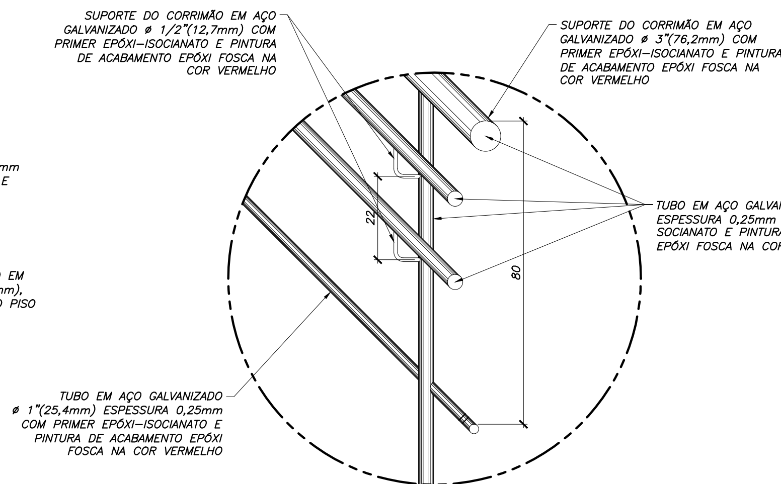
GUARDA-CORPO COM CORRIMÃO ESC. 1:10
