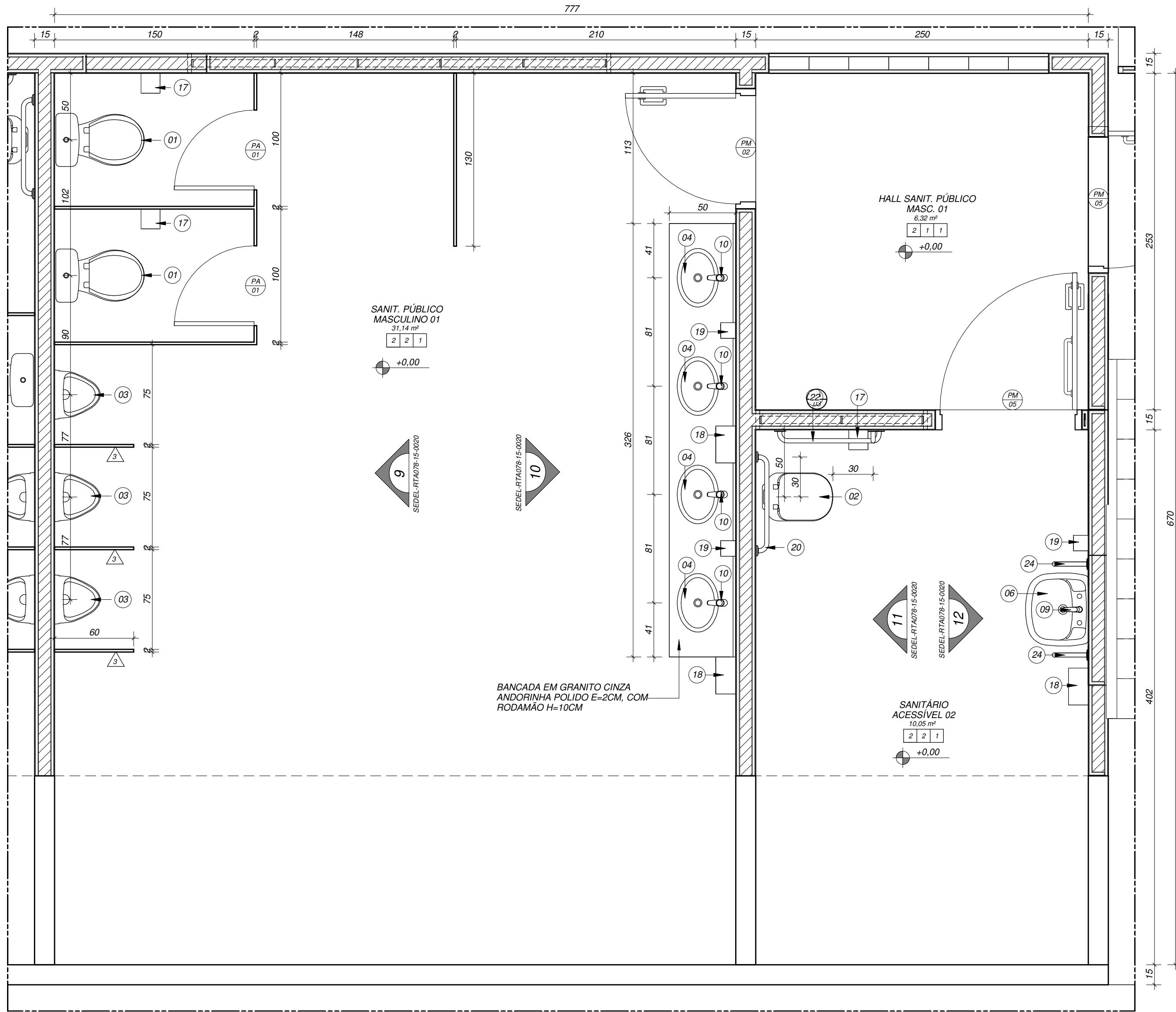
DET.08 - PLANTA BAIXA - SANITÁRIO PÚBLICO MASCULINO 01 1 : 25
