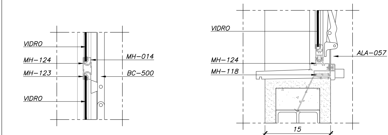
TRECHO CENTRAL ESC. 1:5 DET. GERAIS JANELAS - BASCULANTE ESC. 1:5
