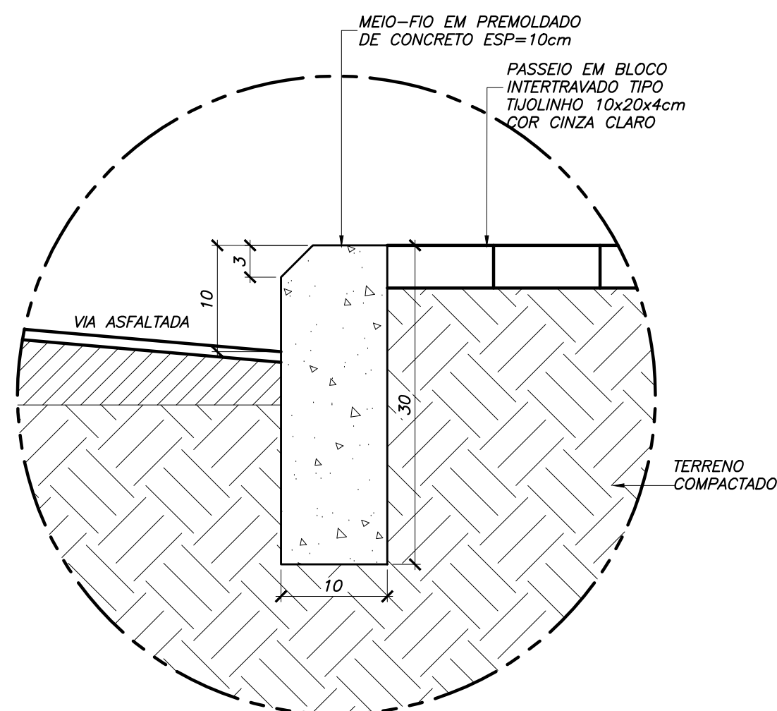
DET. MEIO-FIO ESC. 1:5
