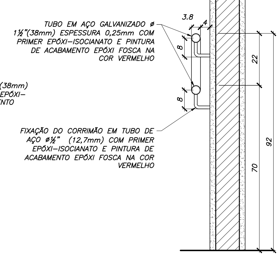
DETALHE CORRIMÃO EM PAREDE ESC. 1:10
