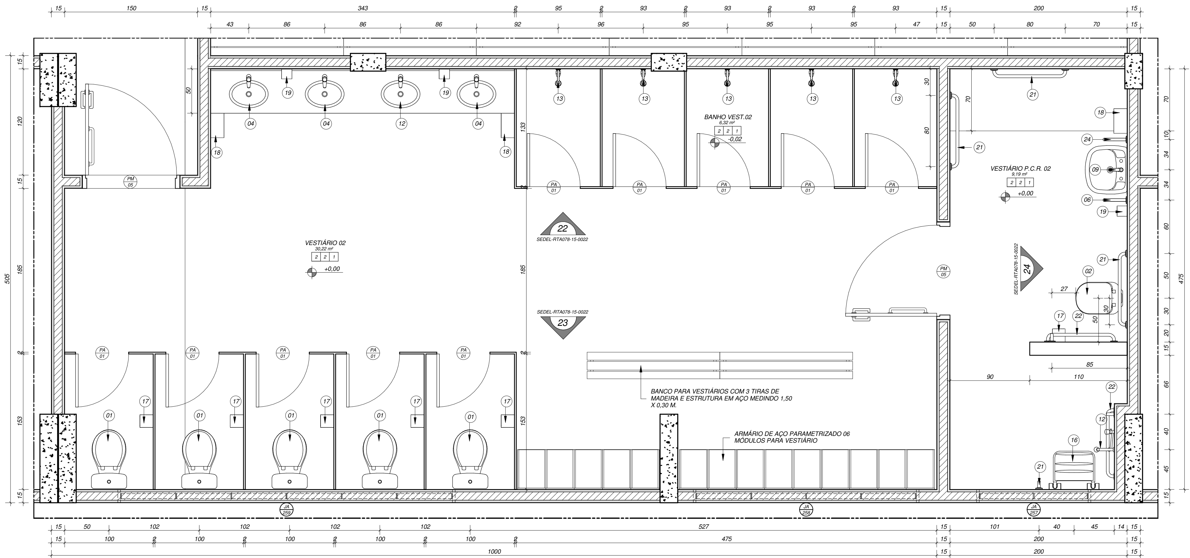
DET.11 - PLANTA BAIXA - VESTIÁRIOS 01/02
