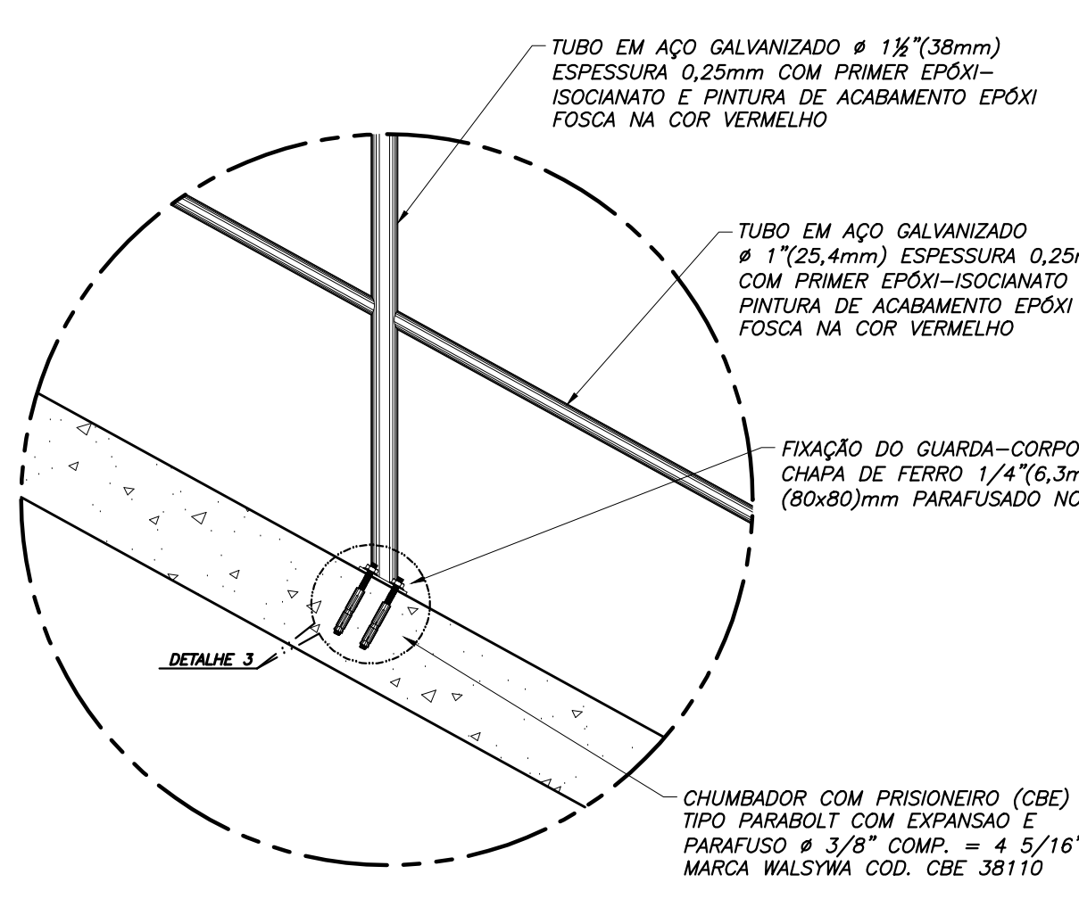
DETALHE 2 ESC. 1:10
