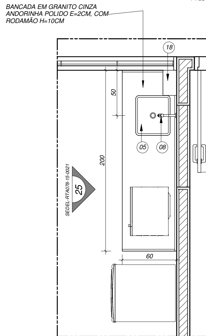
DET.10 - PLANTA BAIXA - COPA
