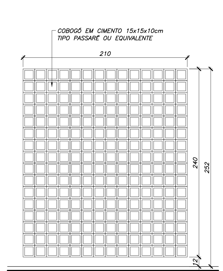
ELEMENTO VAZADO EV-02
