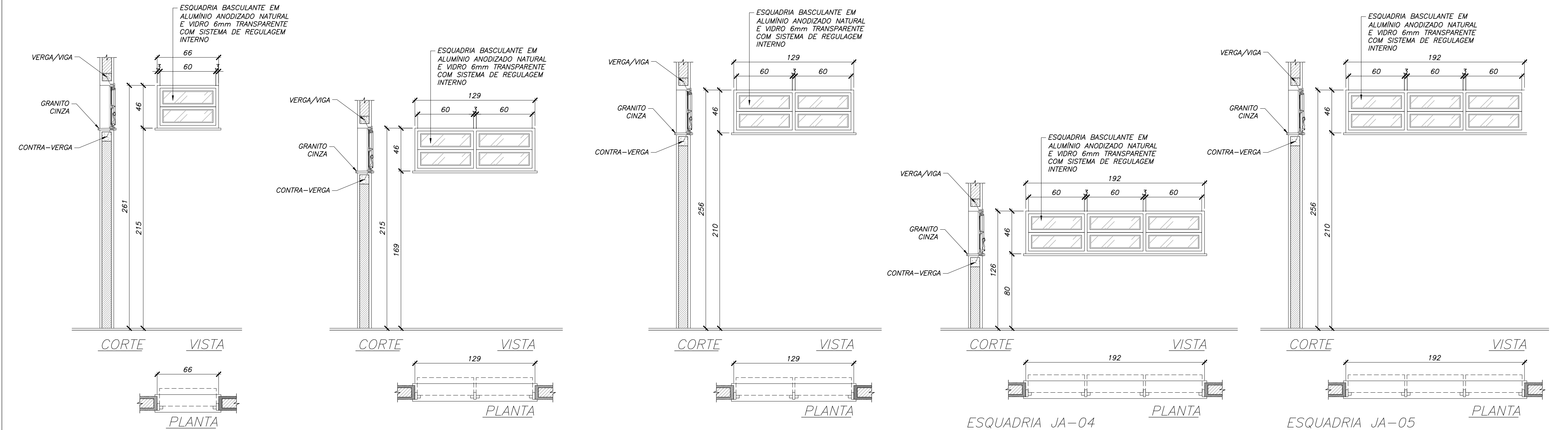
ESQUADRIA JA-01 ESC. 1:25 - QUANTIDADE - 01 UND - SANITÁRIO ACESSÍVEL 04
