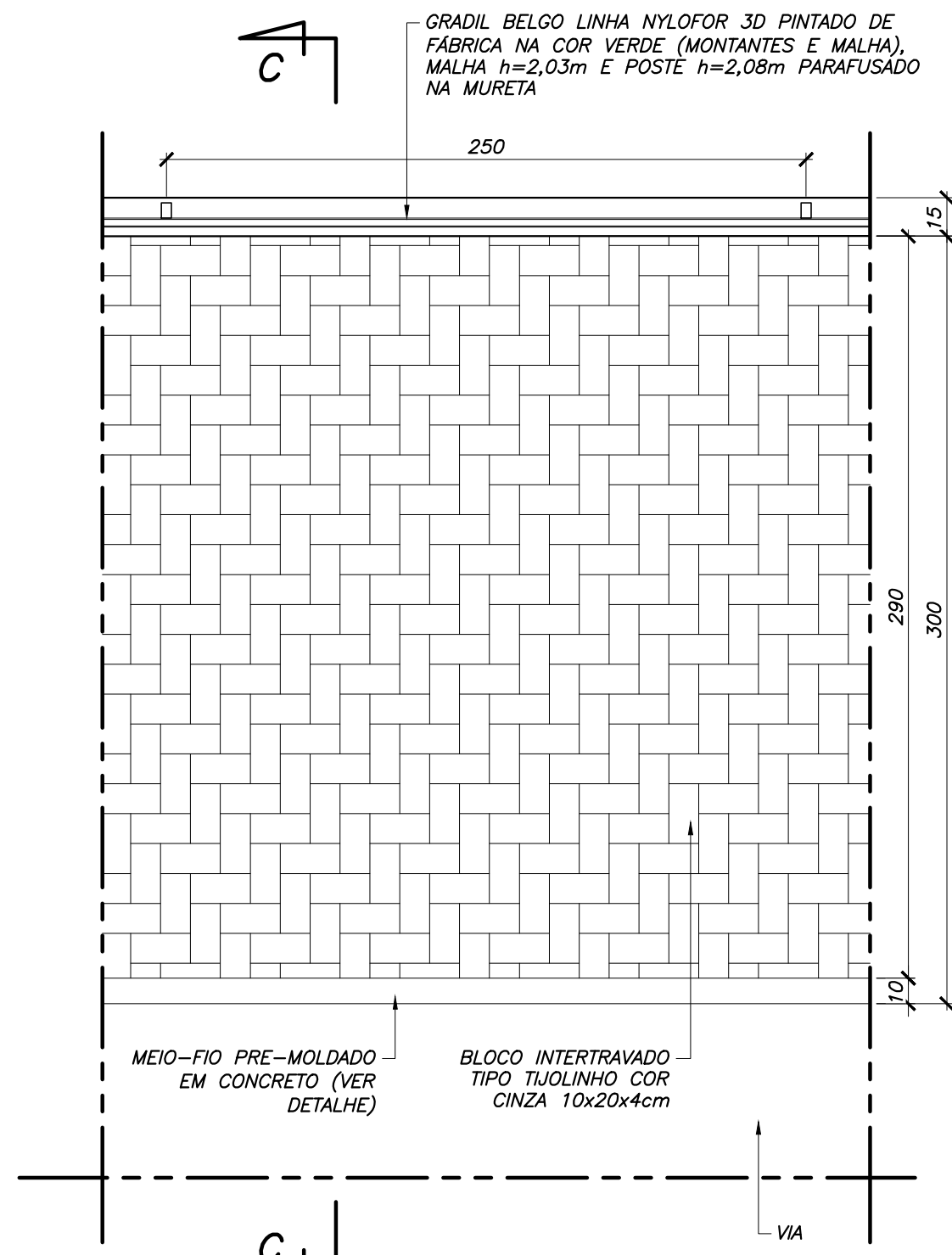
DETALHE DE PASSEIO E GRADIL PERIMETRAL ESC. 1:25
