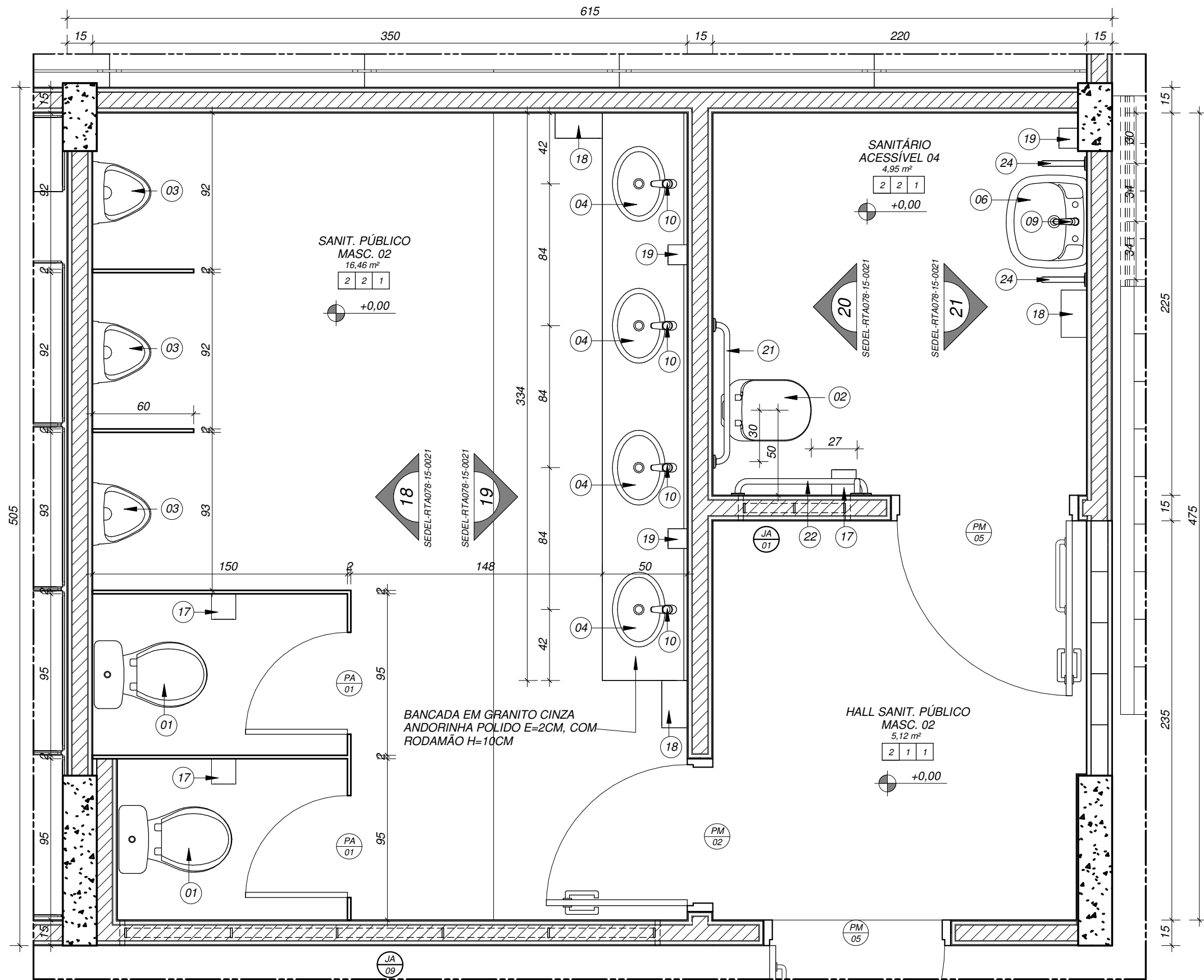
DET.09 - PLANTA BAIXA - SANITÁRIO PÚBLICO MASCULINO 02
