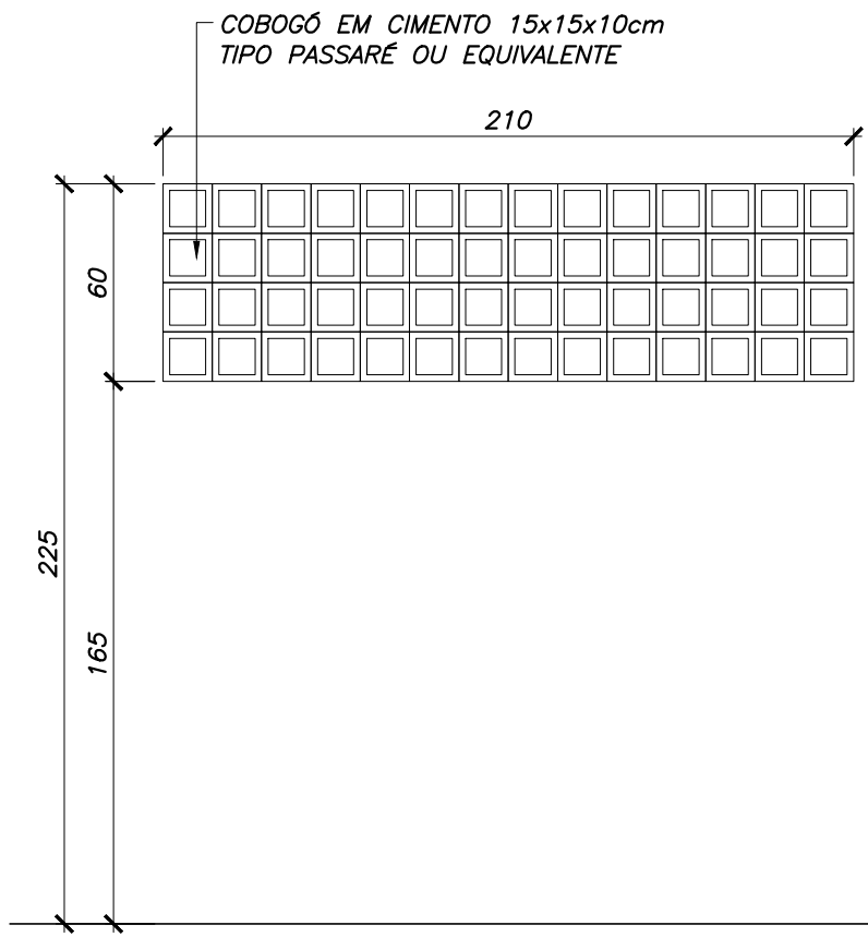
ELEMENTO VAZADO EV-08
