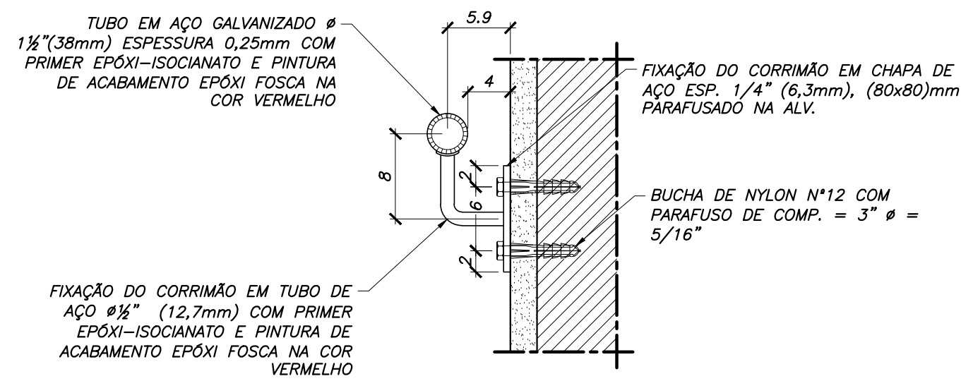
FIXAÇÃO CORRIMÃO DE PAREDE ESC. 1:5
