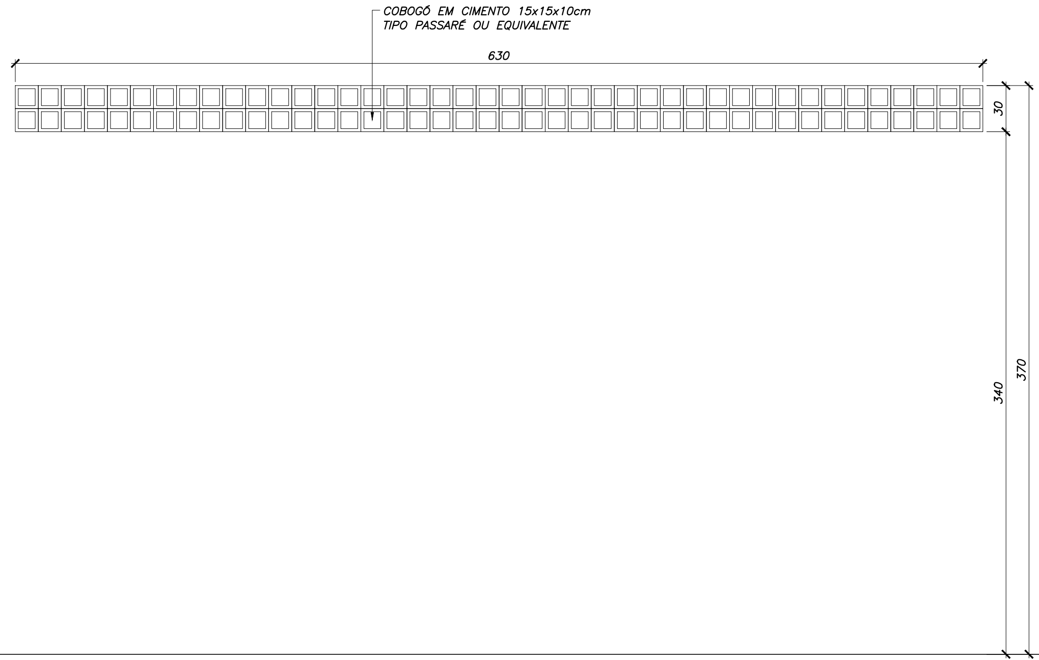
ELEMENTO VAZADO EV-05
