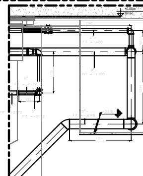
DETALHE B-B
