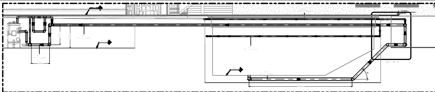
CORTE E-E
