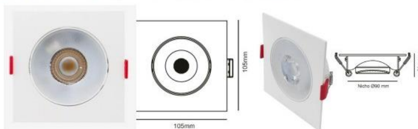
Item 5: SPOT DE EMBUTIR QUADRADO 7W 3000 K (REF. OPUS ECO 33037)
