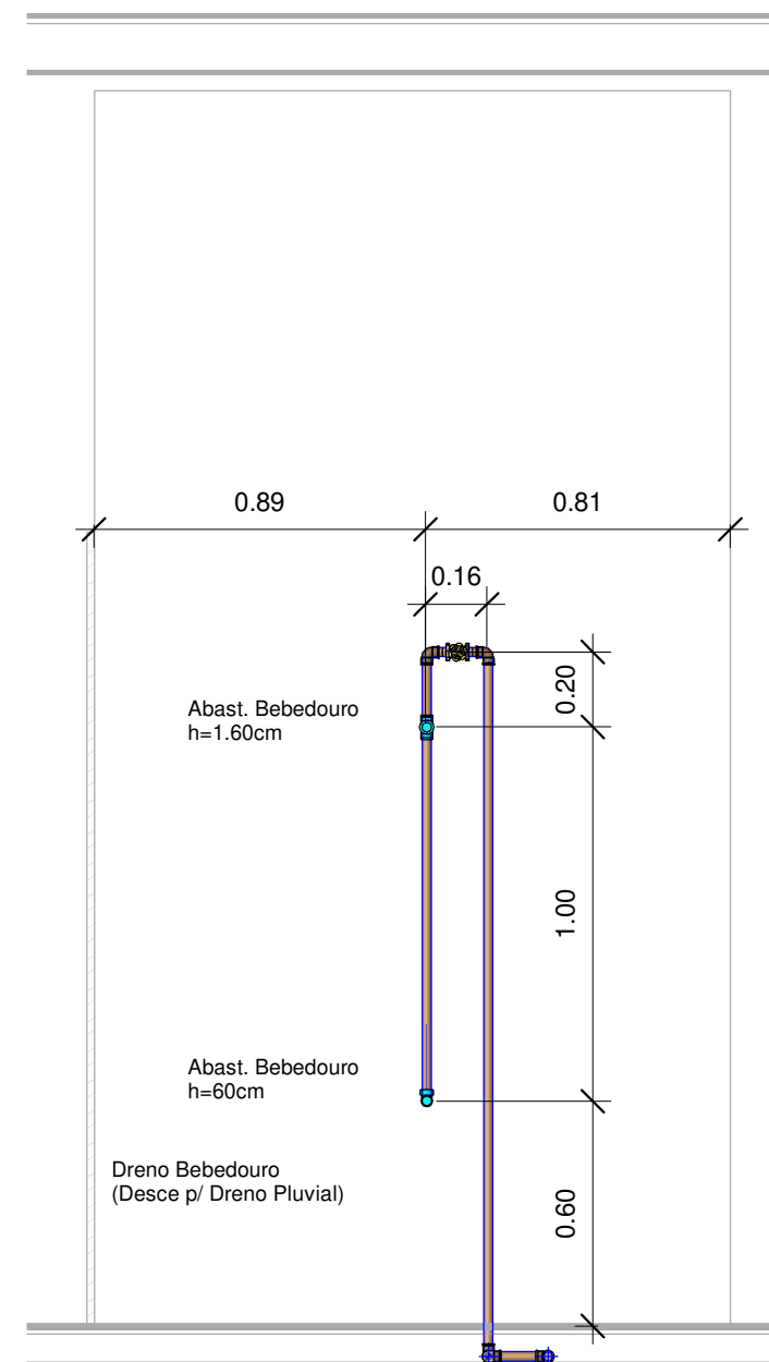
2 BB 1 : 20
