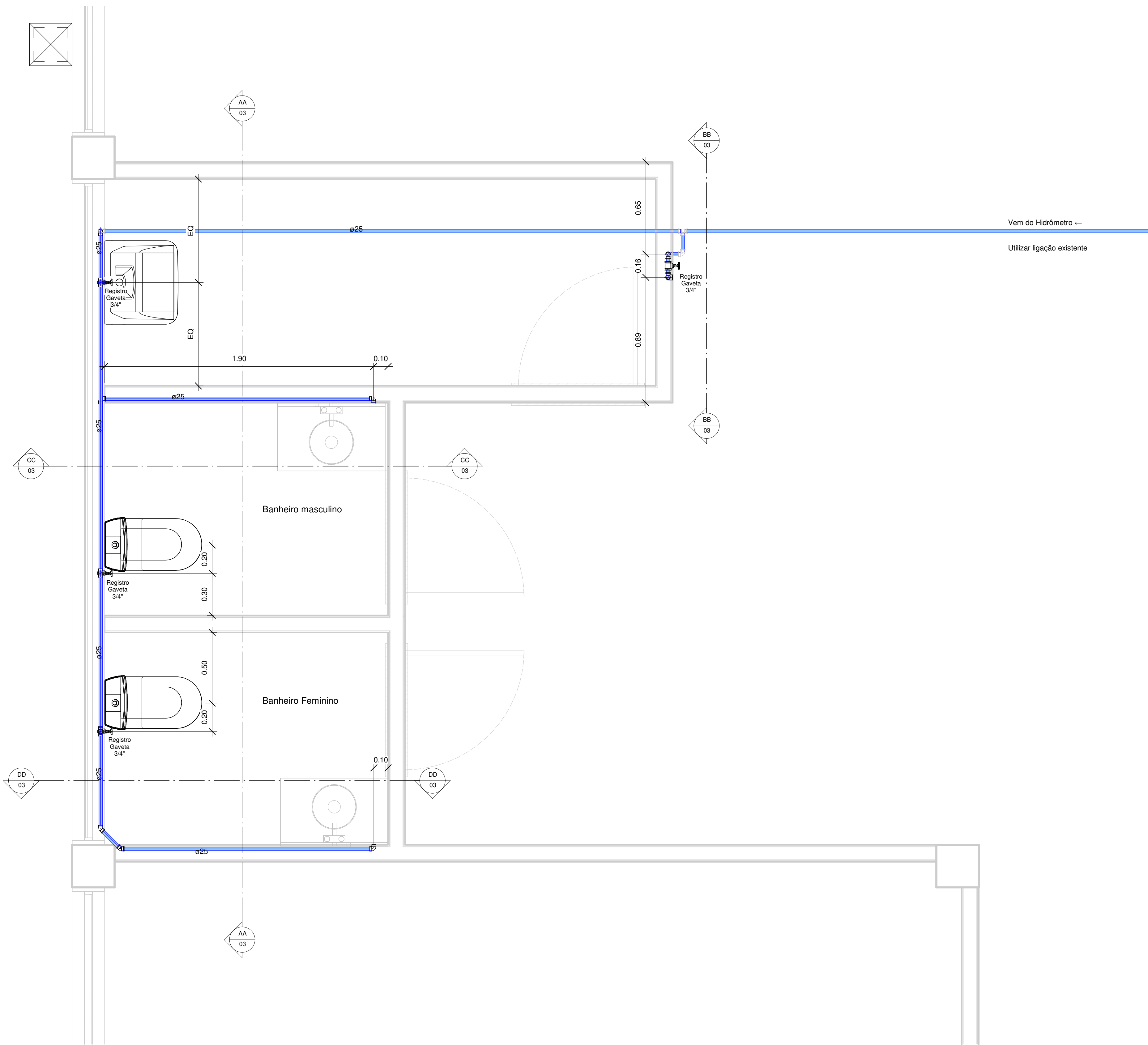
1 Instalações Hidráulicas 1 : 15
