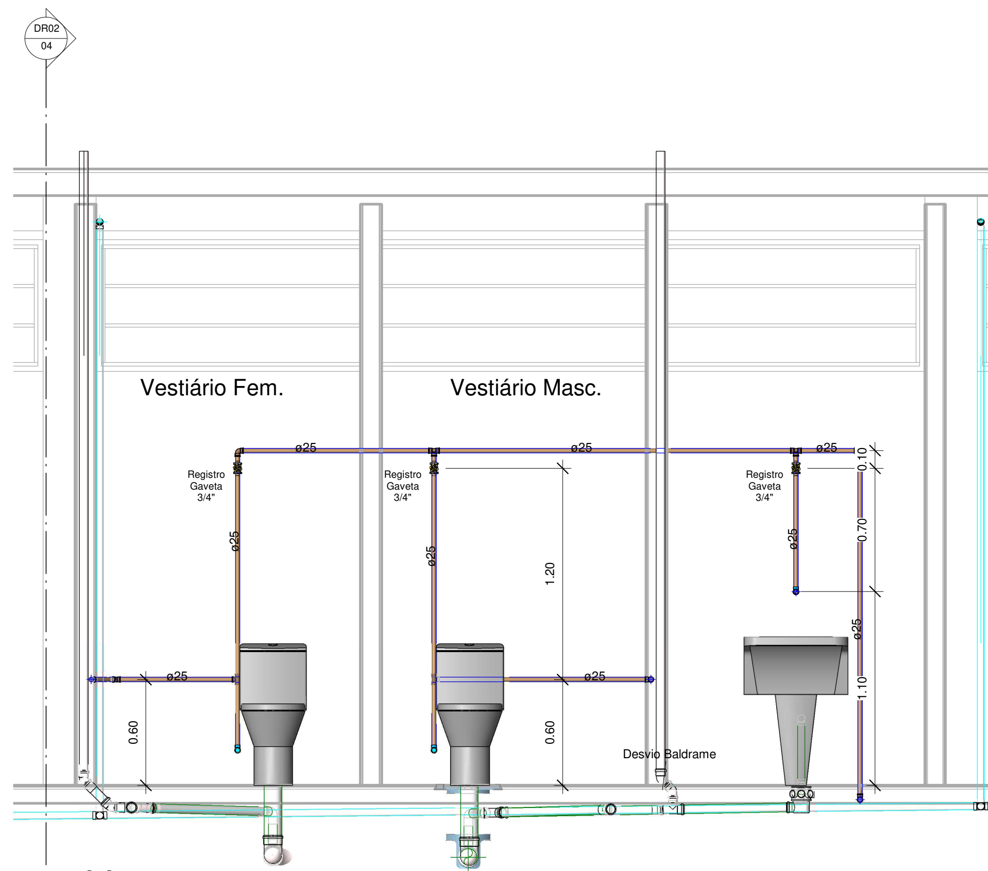
1 AA 1 : 20
