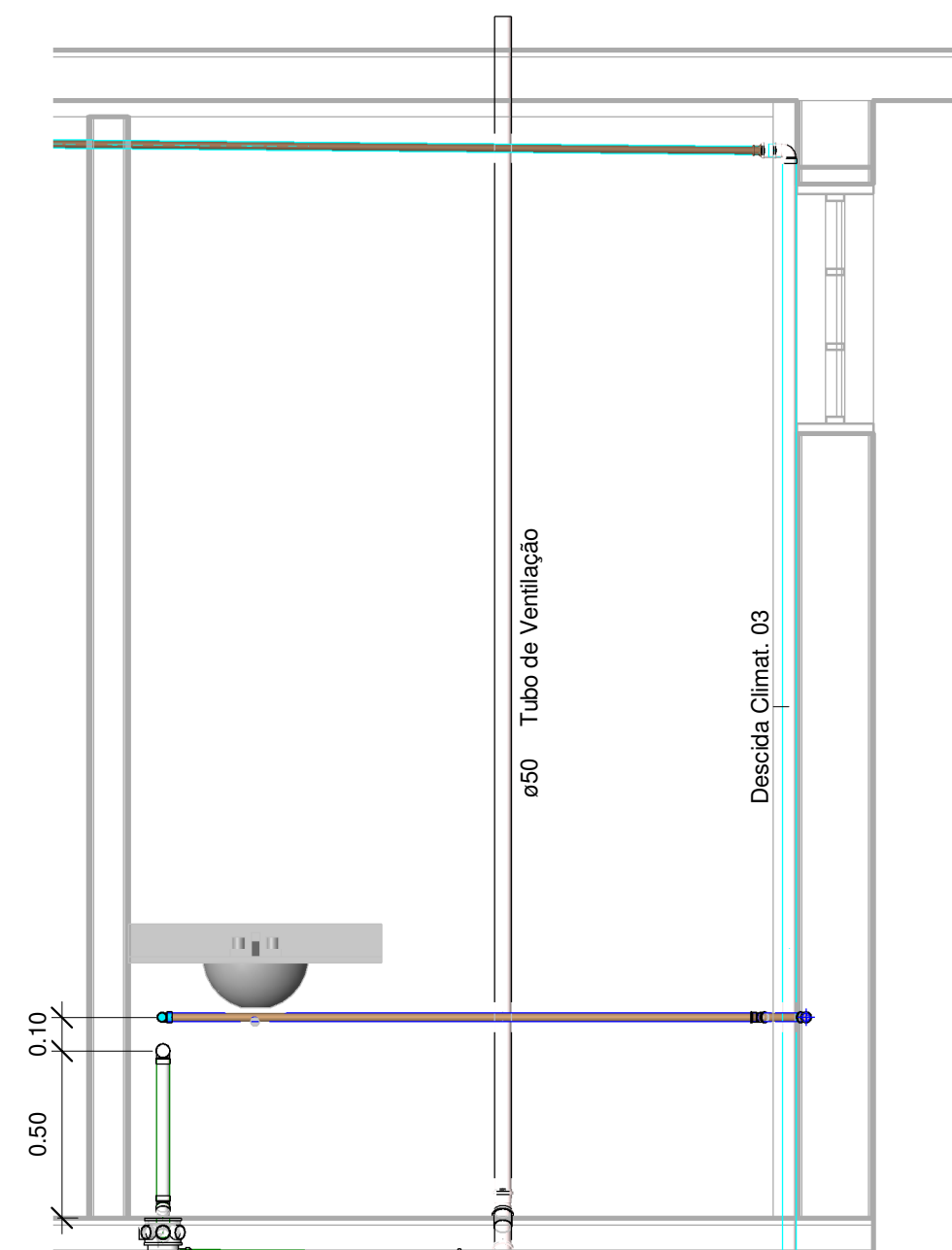
4 DD 1 : 20
