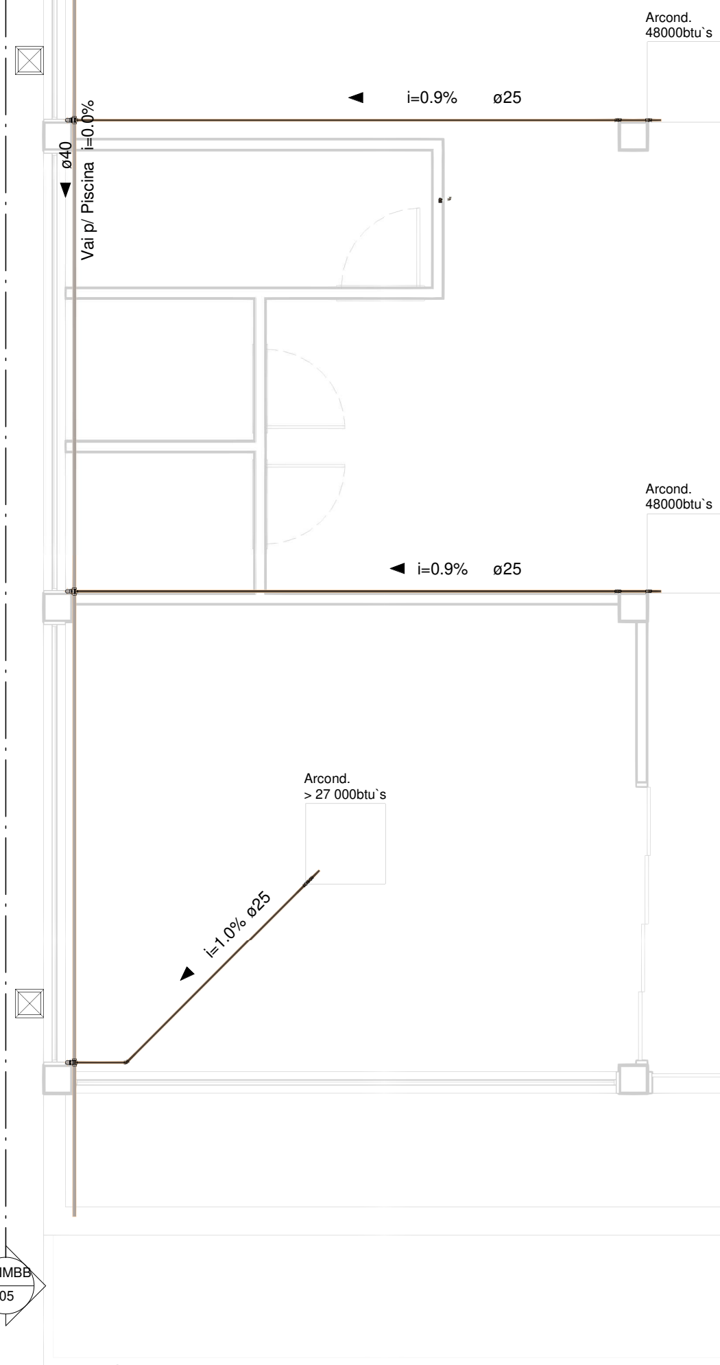
1 Planta Baixa - CLIMAT 1 : 50
