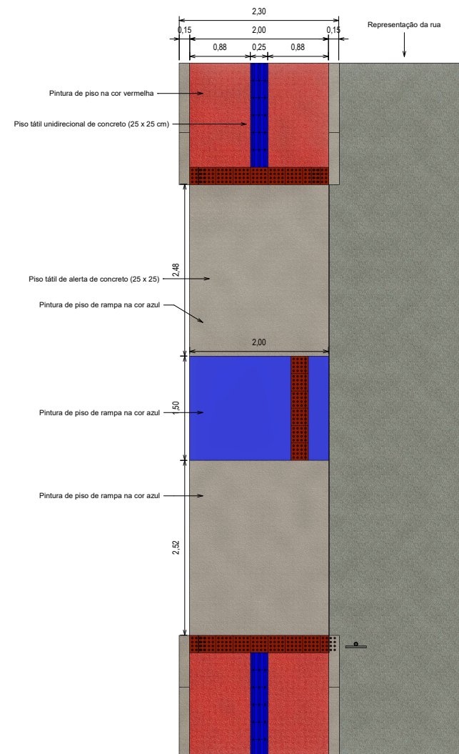
② SEÇÃO TIPO 1 : 25
