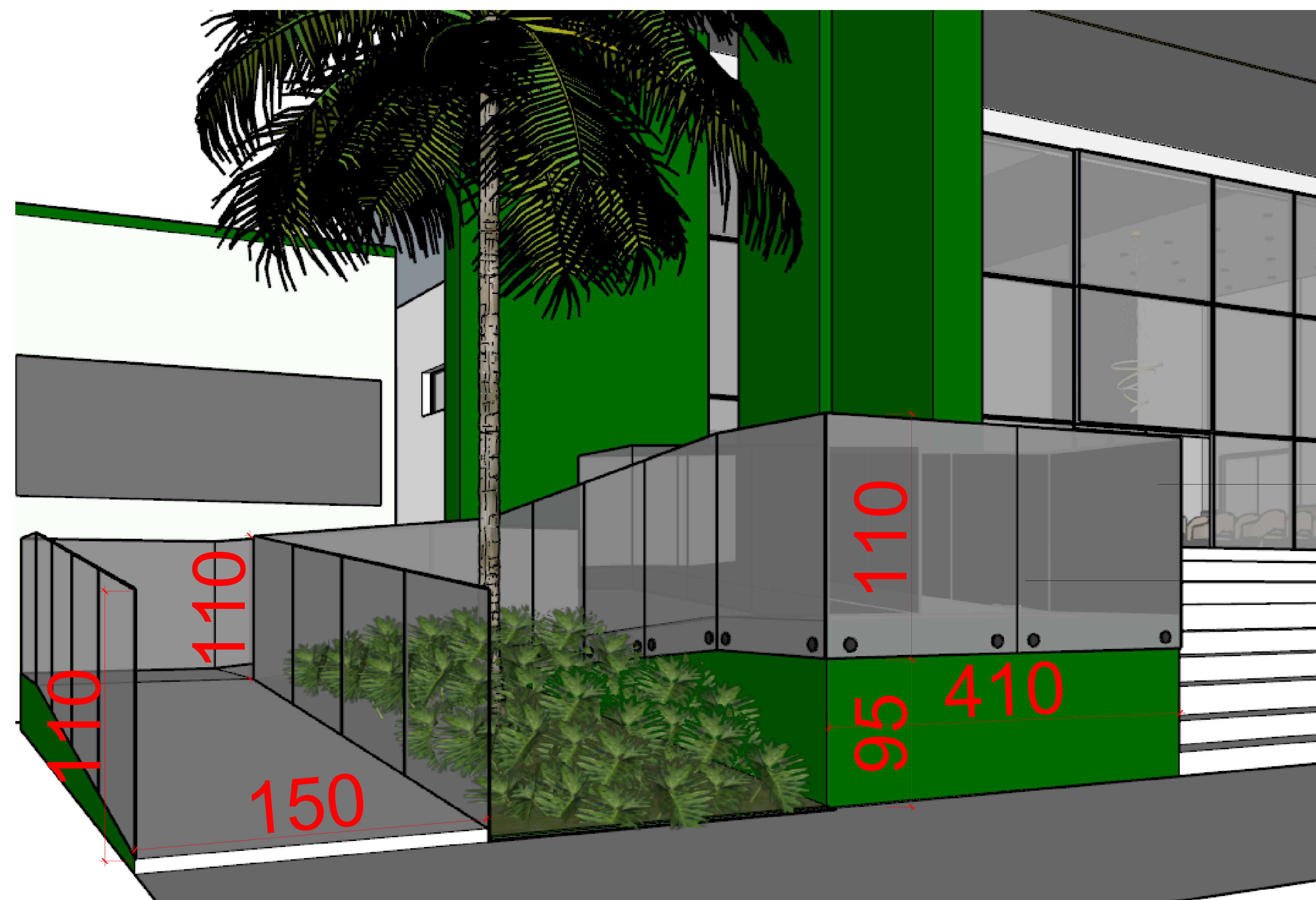
GUARDA CORPO EM VIDRO EXTRA CLEAR FIXADO POR PINÇA
