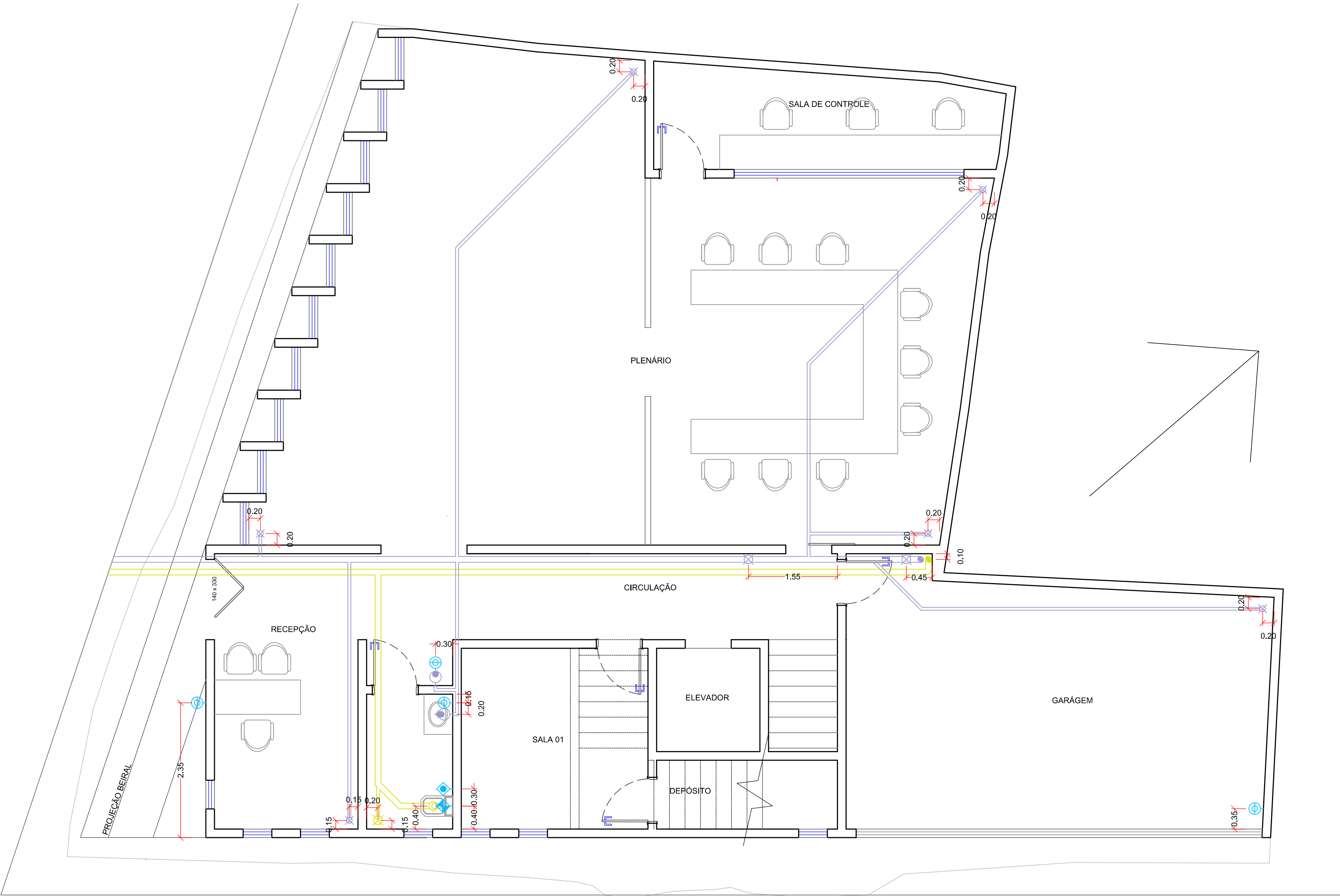
PLANTA DE PONTOS HIDRÁULICOS - TÉRREO ESCALA: 1/50
