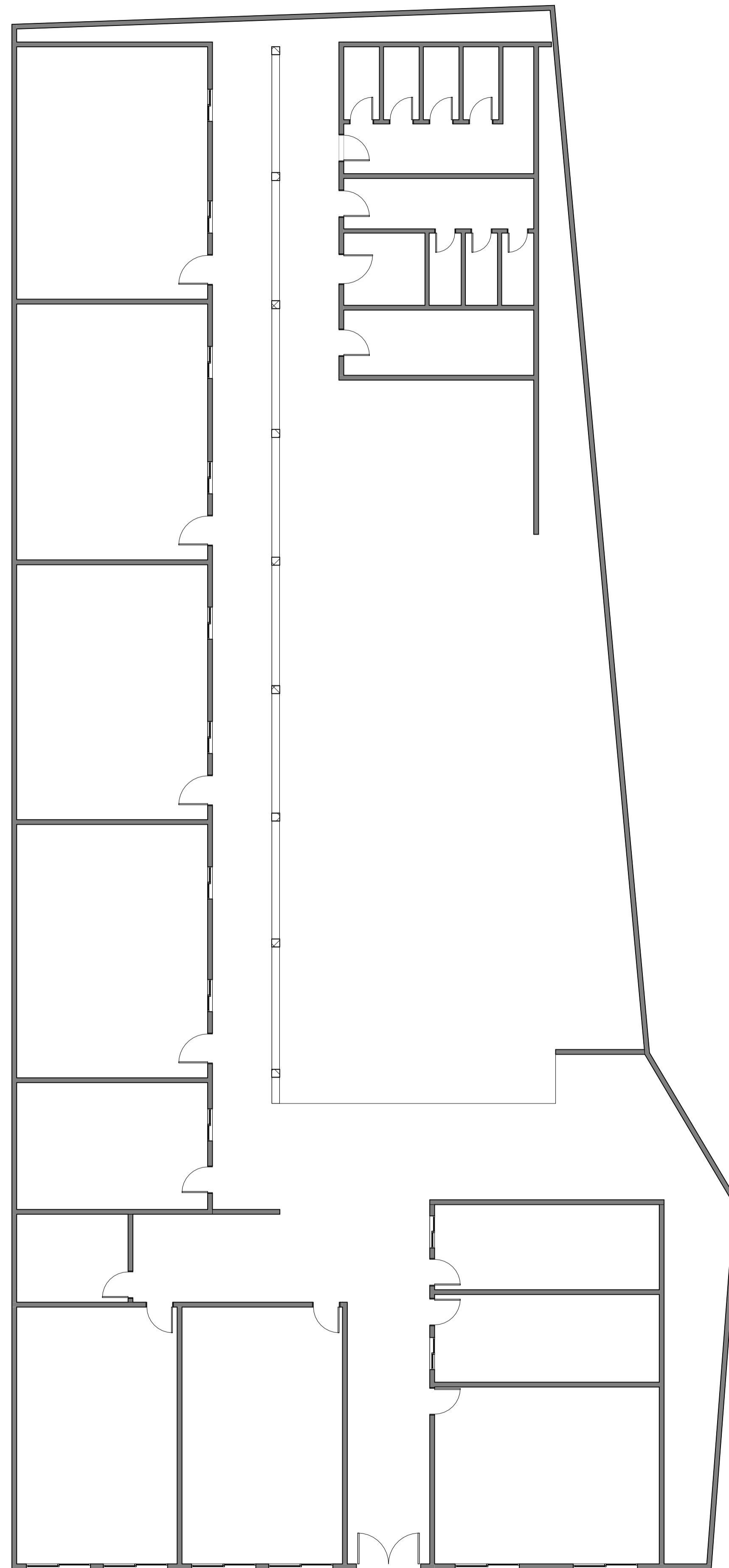
1 Planta baixa - Existente 1 : 100
