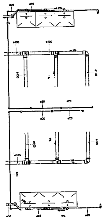
Detalhe - Banheiros 2 Masc./Fem ————— 1:25
