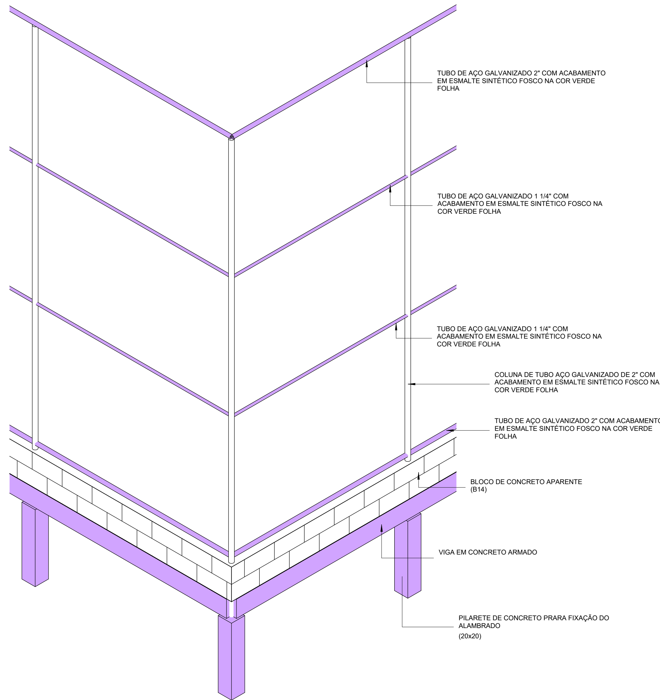
DETALHE-3D_01 ESCALA
