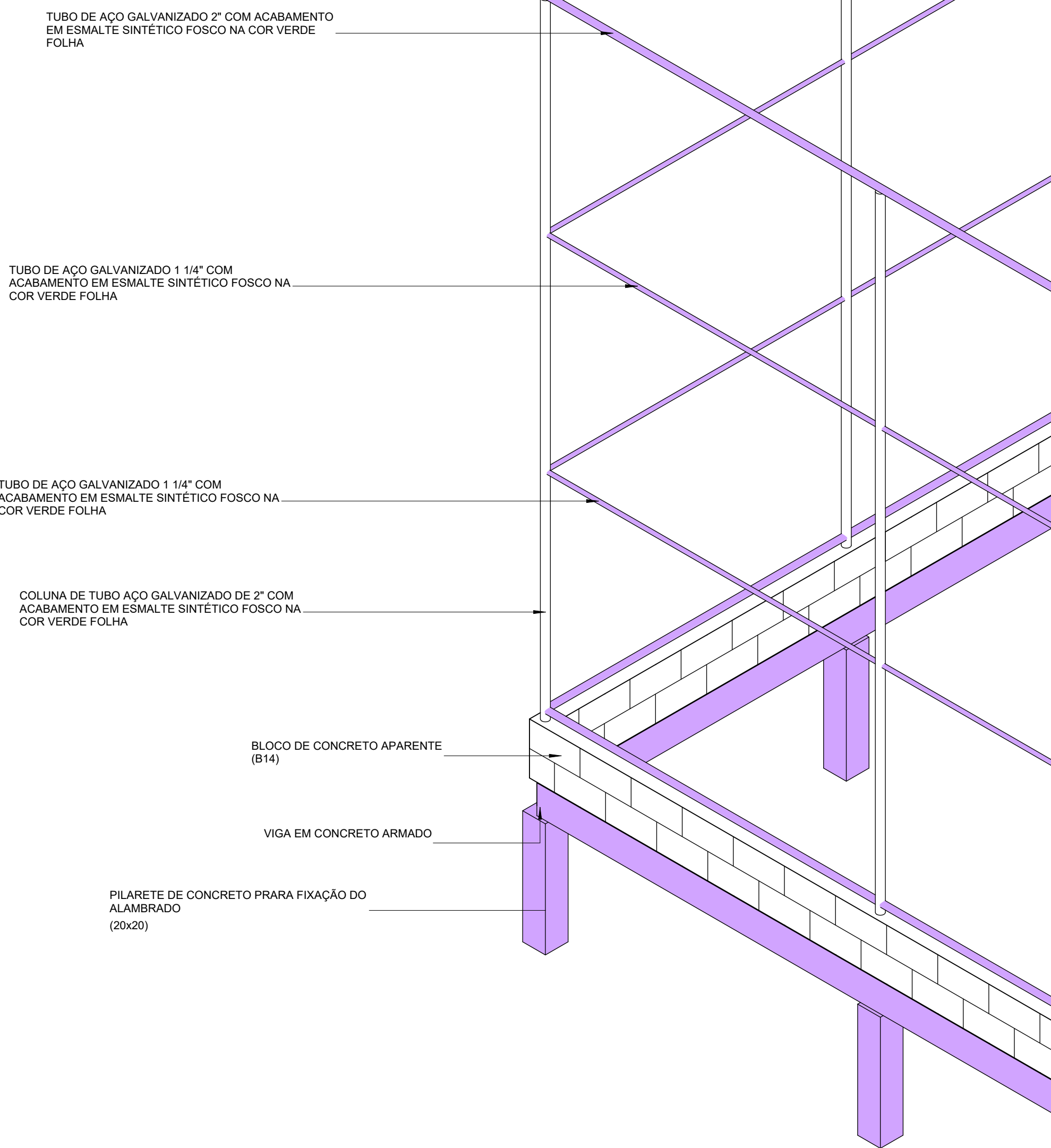
DETALHE-3D_02 ESCALA
