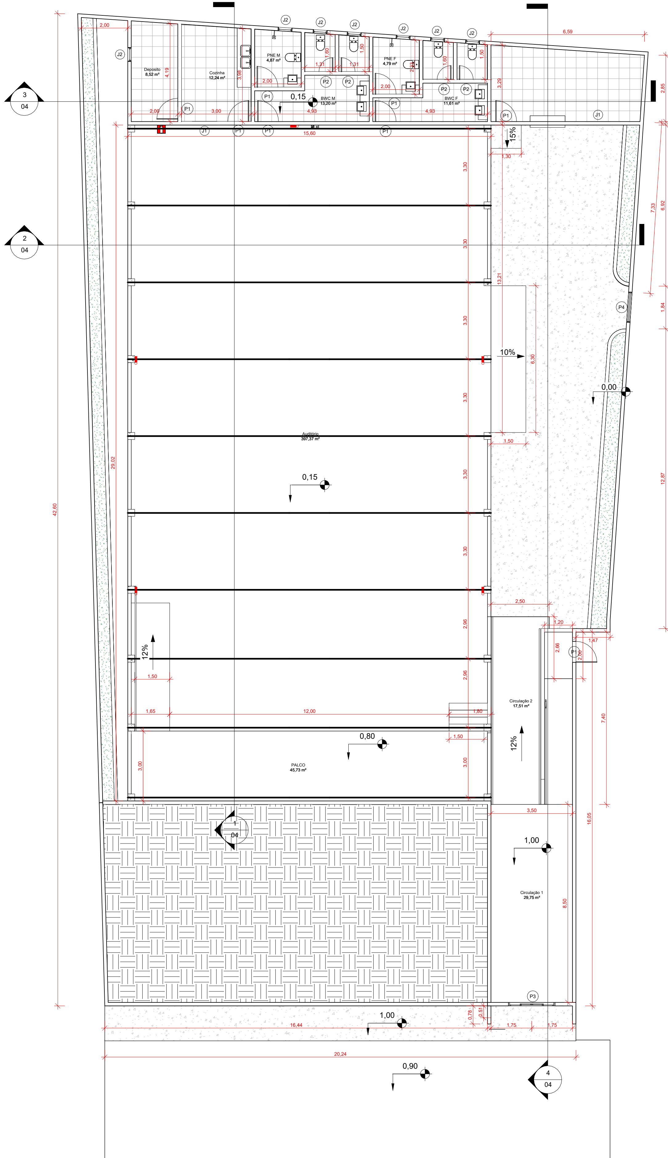
1 PLANTA BAIXA TÉRREO 1 : 100
