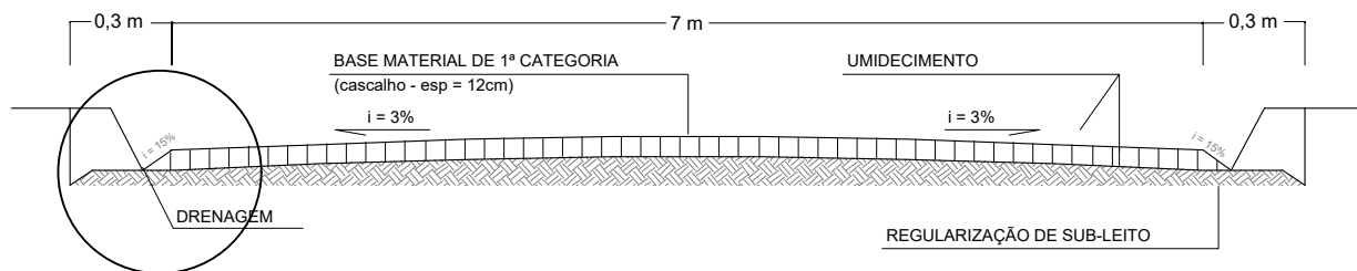
SARJETA SEM REVESTIMENTO COM SEÇÃO TRIANGULAR 88-20
