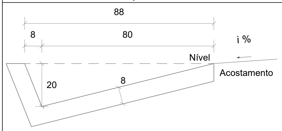
SEÇÃO TRANSVERSAL - SARJETA SEM REVESTIMENTO
