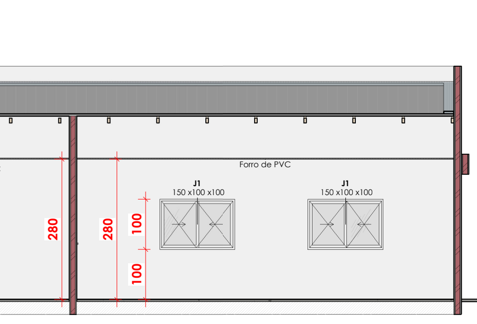
7 Lateral esquerda 1 : 75
