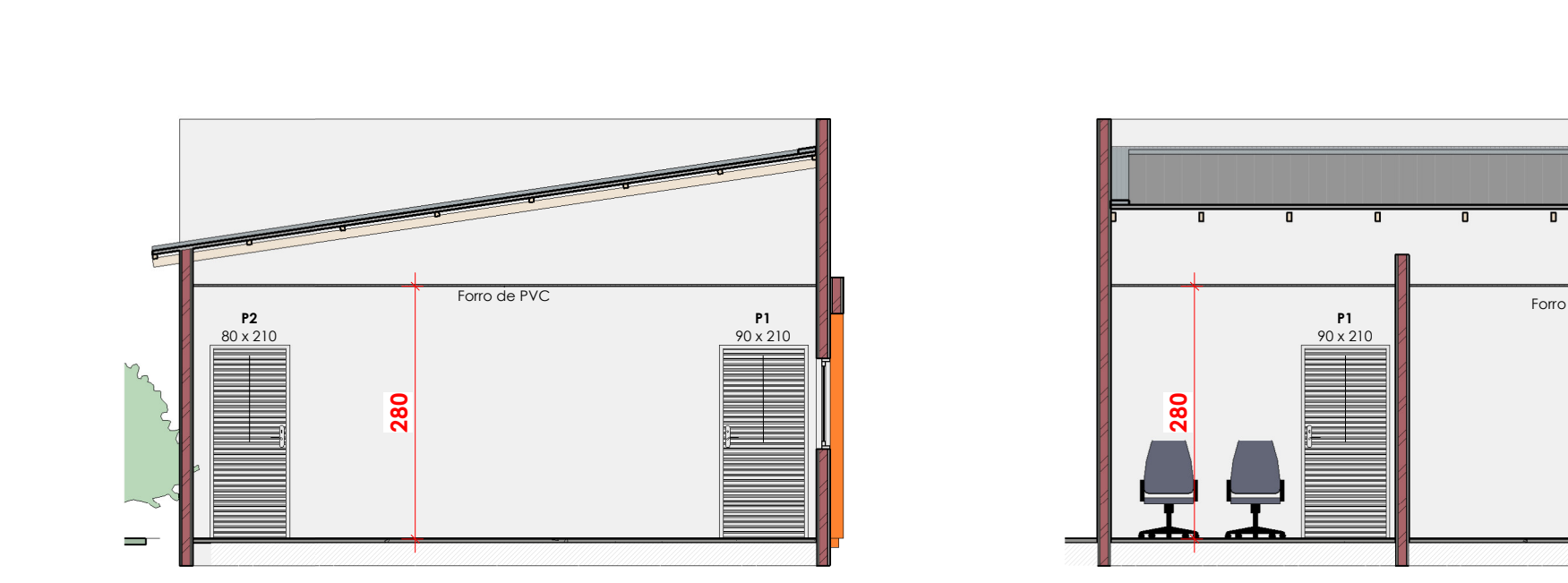
18 BB 1 : 75
