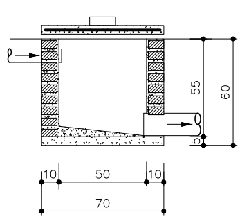
CORTE AA
