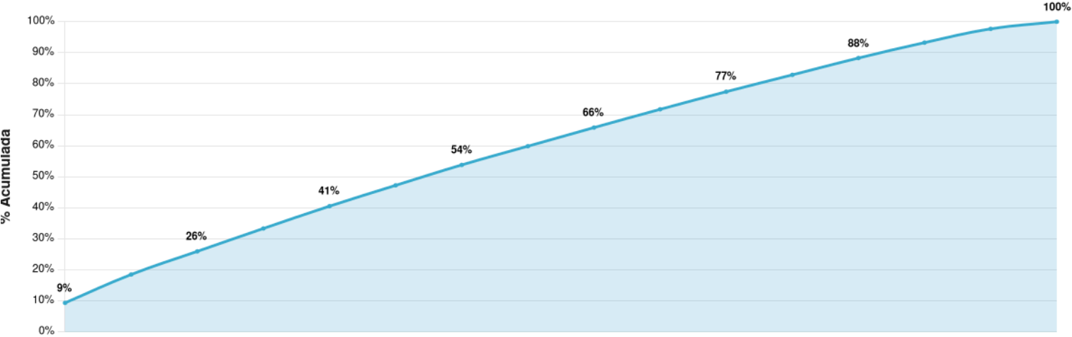
Curva ABC
