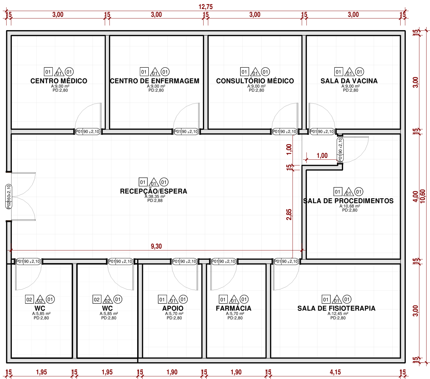
1 TÉRREO - ESCALA 1 : 75
