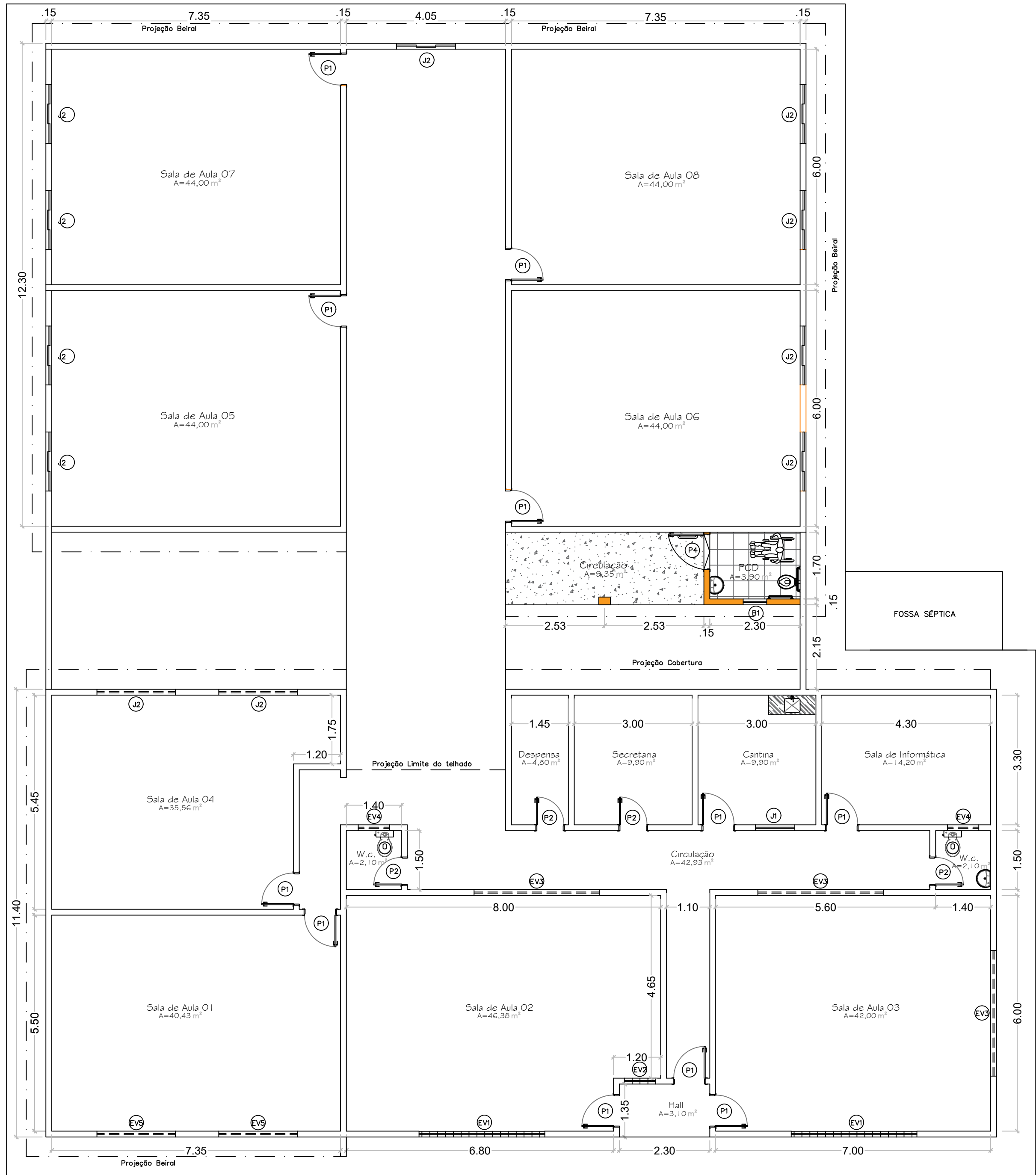
01 PLANTA BAIXA DE INTERVENÇÃO Esc: 1/75
