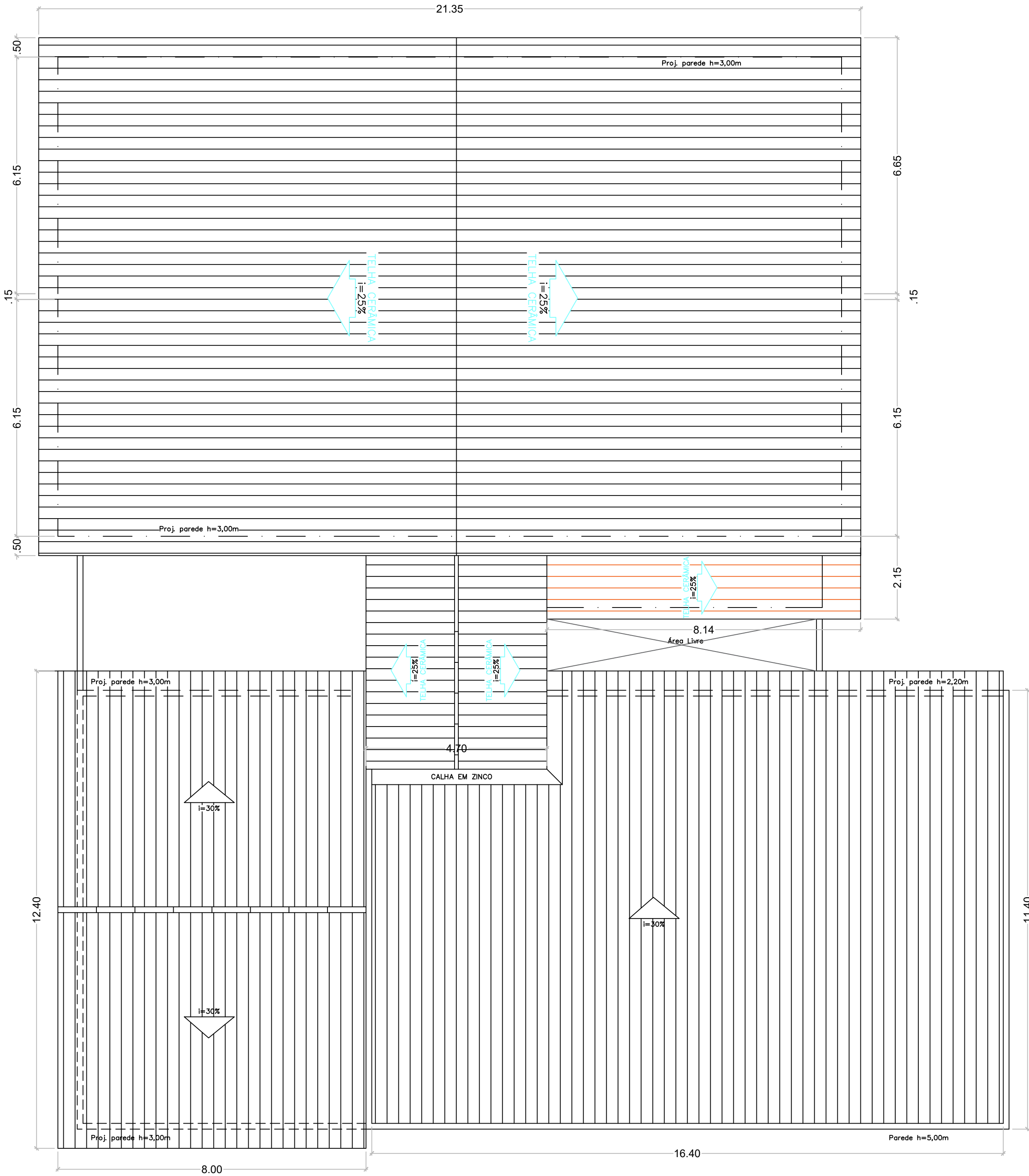
02 PLANTA DE COBERTURA Esc: 1/75
