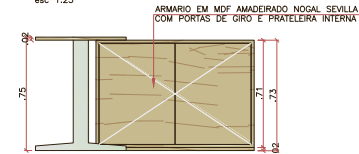
M-01 - DETALHAMENTO - VISTA 03 esc 1:25
