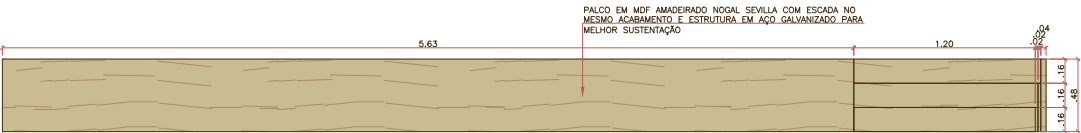
M-11 - DETALHAMENTO - VISTA 1
