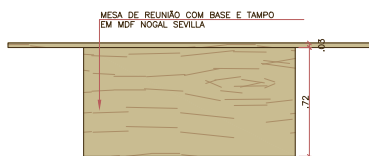
M-09 - DETALHAMENTO - VISTA 01 esc 1:25
