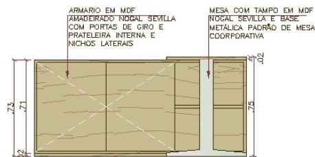
M-07 - DETALHAMENTO - VISTA 02 esc 1:25
