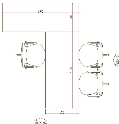
M-07 - DETALHAMENTO - PLANTA BAIXA esc 1:25
