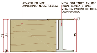
M-01 - DETALHAMENTO - VISTA 01 esc 1:25
