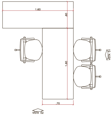
M-07 - DETALHAMENTO - PLANTA BAIXA esc 1:25
