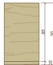
M-05 - DETALHAMENTO - VISTA 02 esc 1:25
