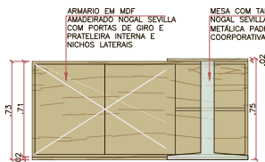
M-07 - DETALHAMENTO - VISTA 02 esc 1:25
