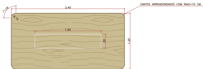
M-09 - DETALHAMENTO - PLANTA BAIXA esc 1:25
