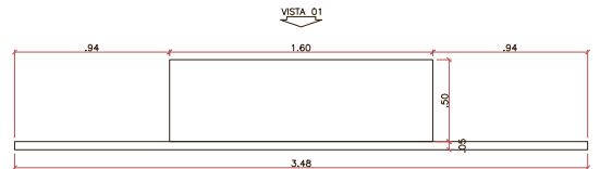
M-08 - DETALHAMENTO - VISTA 01 esc 1:25
