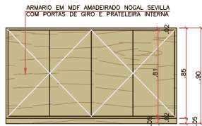
M-05 - DETALHAMENTO - VISTA 01 esc 1:25
