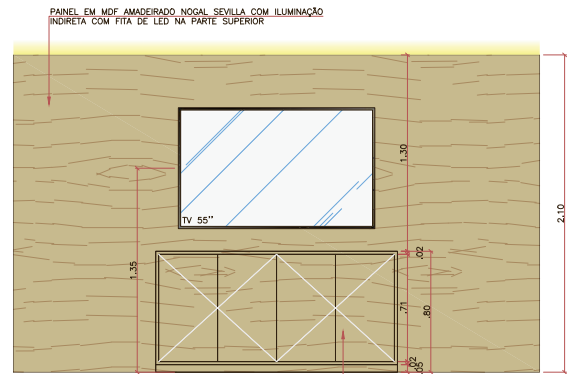
M-08 - DETALHAMENTO - PLANTA BAIXA esc 1:25
