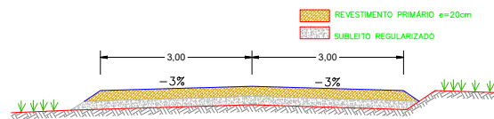
SEÇÃO TIPO DO REVESTIMENTO PRIMÁRIO e=20cm S/ ESCALA TODOS OS TRECHOS
