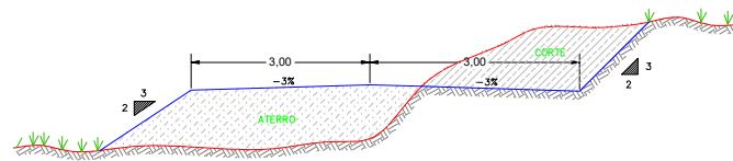
SEÇÃO TIPO DE TERRAPLENAGEM S/ ESCALA TODOS OS TRECHOS
