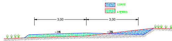
SEÇÃO TIPO DO REGULARIZAÇÃO DO SUBLEITO S/ ESCALA TODOS OS TRECHOS
