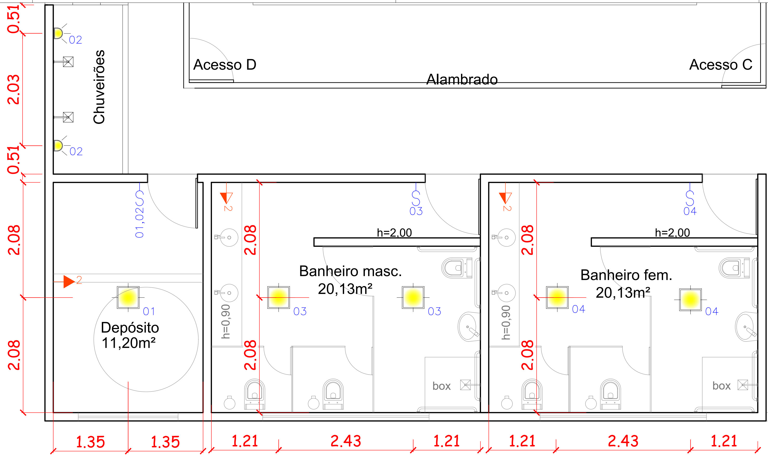
PLANTA BAIXA LUMINOTÉCNICA WC'S/DEPÓSITO ESCALA 1/25
