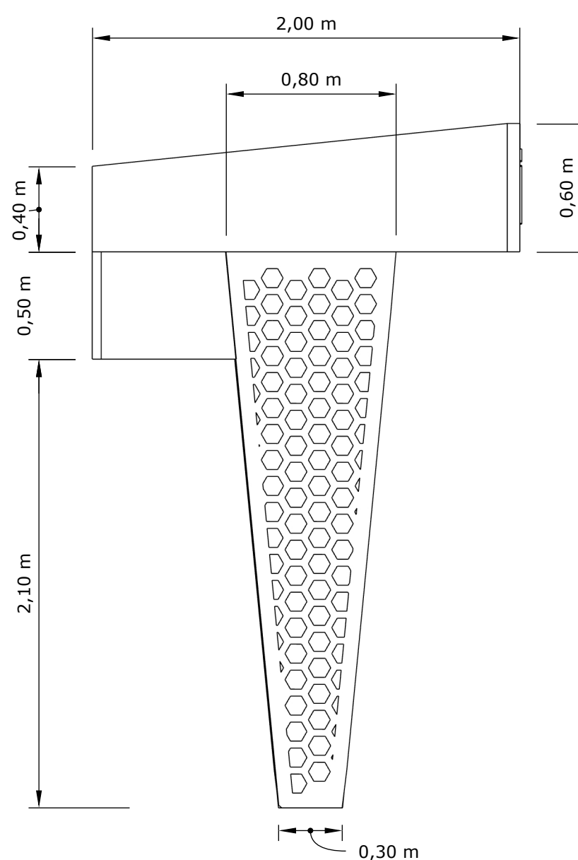
3 VISTA LATERAL ESQUERDA ESCALA: 1:50
