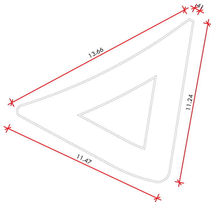
02 PLANTA TÉCNICA - TRIÂNGULO 02 ESCALA: 1 | 150
