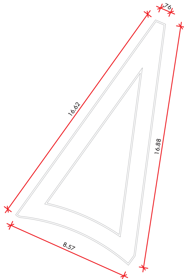
01 PLANTA TÉCNICA - TRIÂNGULO 01 ESCALA: 1 | 150
