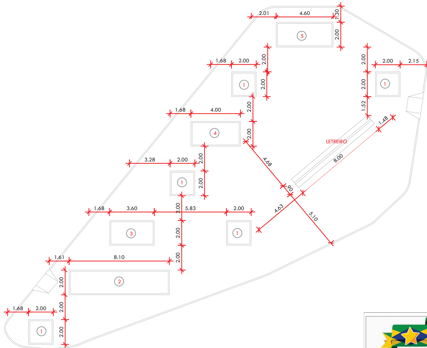
01 | PLANTA DE LOCAÇÃO DE CANTEIROS E LETREIRO ESCALA: 1 | 150
