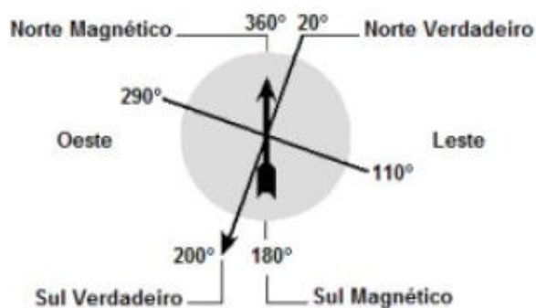
Figura 1 Orientação instalação placas solares
