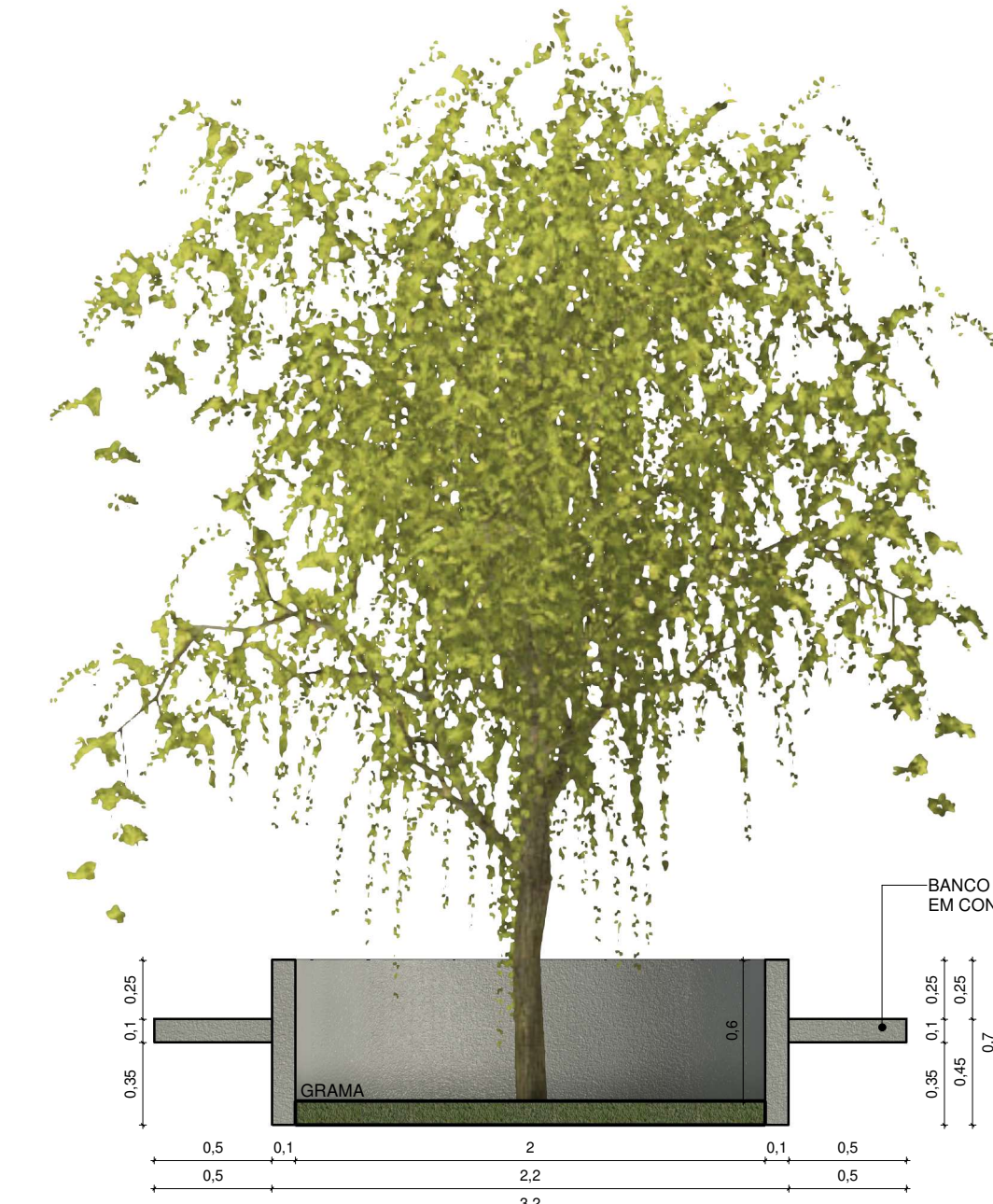
DET.01 - CORTE AA* ESC. 1 : 30
