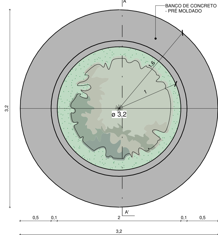
DET.01 - PLANTA BAIXA ESC. 1 : 30
