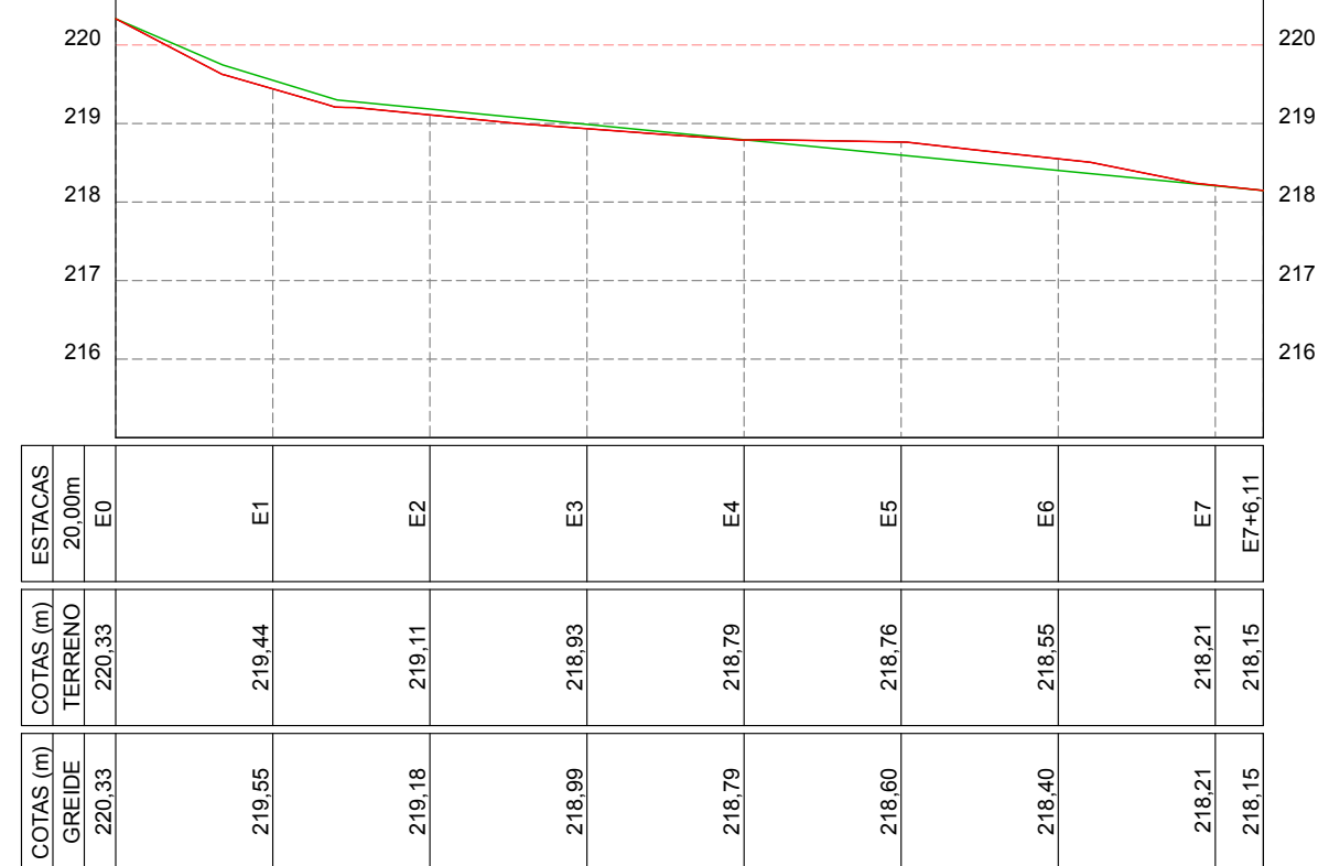
RUA MANOEL FERREIRA ESCALA VERTICAL 1/100 ESCALA HORIZONTAL 1/1000
