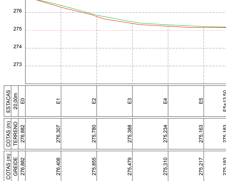
RUA PROJETADA ESCALA VERTICAL 1/100 ESCALA HORIZONTAL 1/1000
