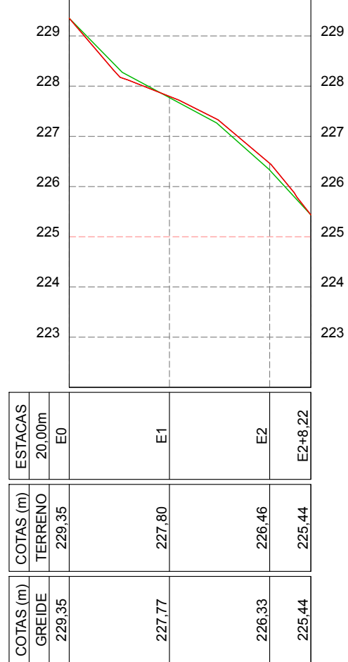
RUA 7 DE SETEMBRO ESCALA VERTICAL 1/100 ESCALA HORIZONTAL 1/1000
