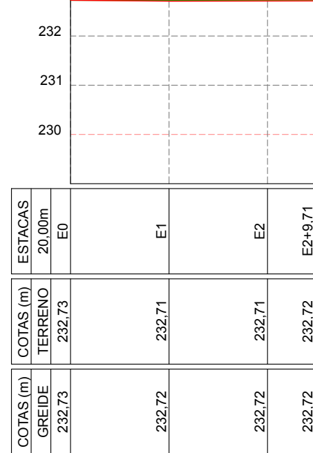
RUA PEDRO RODRIGUES ESCALA VERTICAL 1/100 ESCALA HORIZONTAL 1/1000
