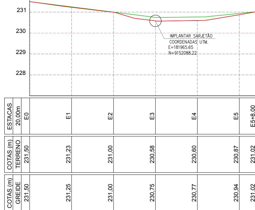
RUA PETRONIO PORTELA ESCALA VERTICAL 1/100 ESCALA HORIZONTAL 1/1000
