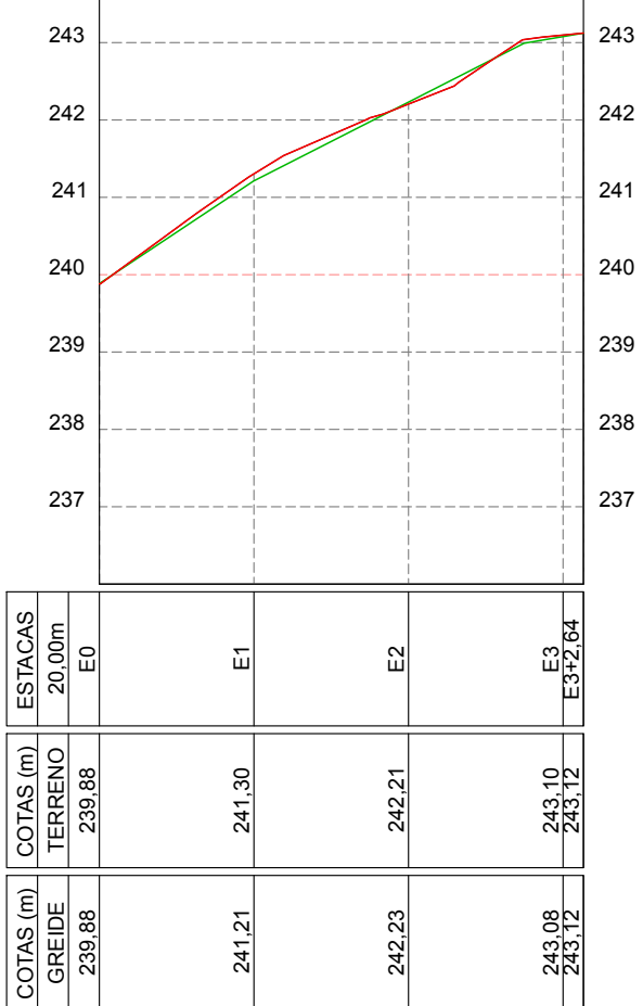
RUA ARISTIDES CESAR DO NASCIMENTO ESCALA VERTICAL 1/100 ESCALA HORIZONTAL 1/1000
