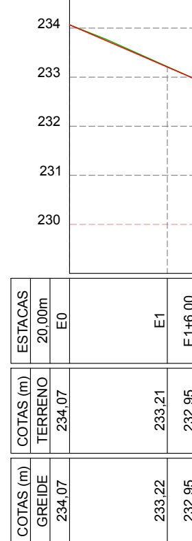
RUA ANTONIO ALVES - TRECHO 01 ESCALA VERTICAL 1/100 ESCALA HORIZONTAL 1/1000
