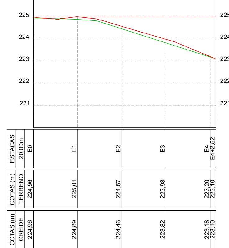
RUA MARTINHO ANTUNES FERREIRA ESCALA VERTICAL 1/100 ESCALA HORIZONTAL 1/1000
