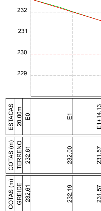
RUA ERMELINDO ALVES DE BARROS ESCALA VERTICAL 1/100 ESCALA HORIZONTAL 1/1000
