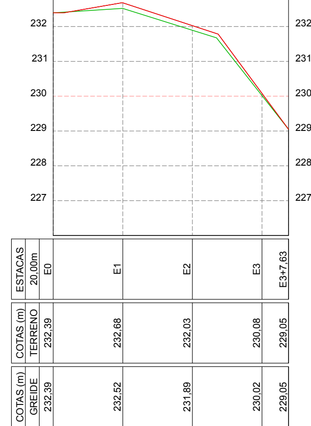
RUA JOÃO PINHEIRO SOBRINHO ESCALA VERTICAL 1/100 ESCALA HORIZONTAL 1/1000
