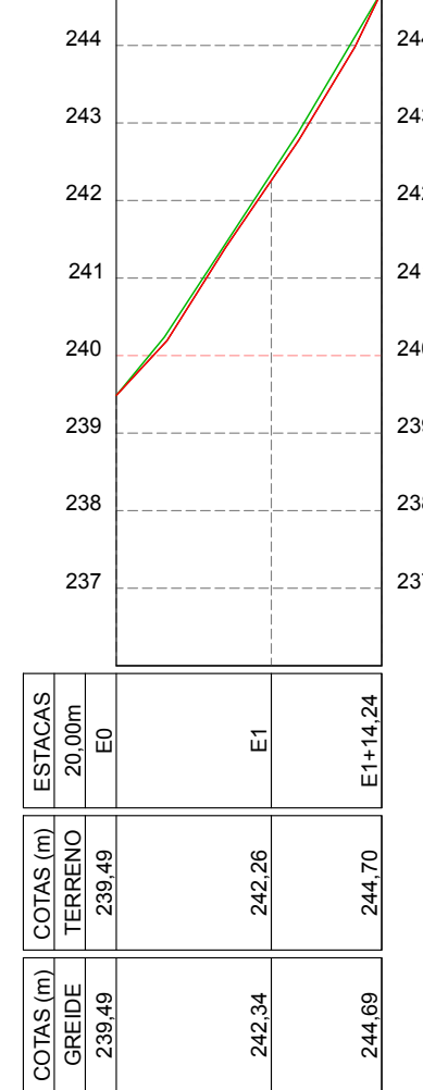
RUA ANTONIO ALVES - TRECHO 02 ESCALA VERTICAL 1/100 ESCALA HORIZONTAL 1/1000
