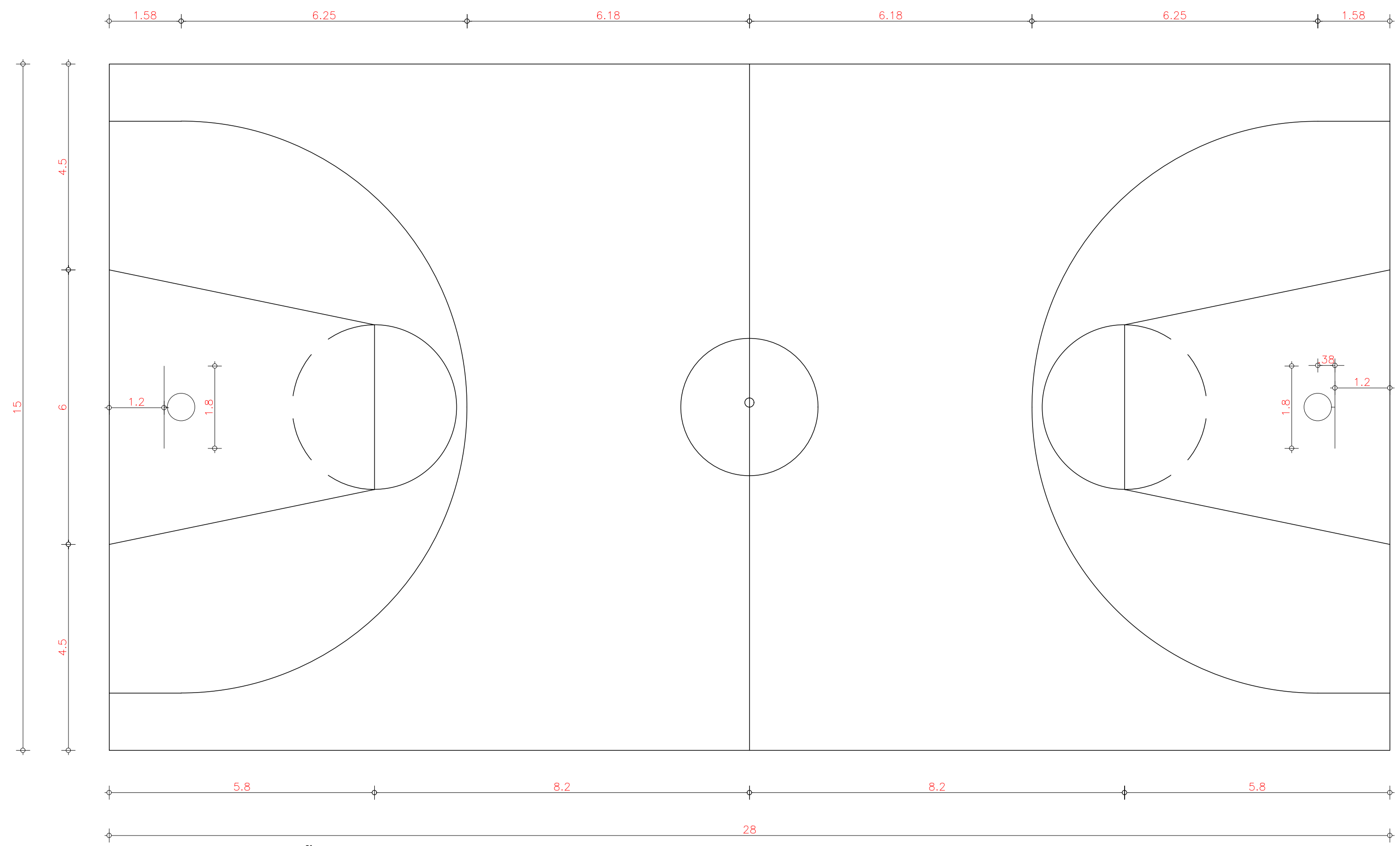
04 DEMARCAÇÃO - BASQUETBOL esc.: 1/75
