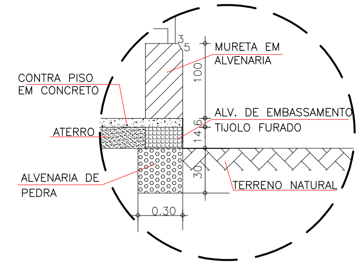
08 DETALHE - 01 E 02 esc.: 1/25
