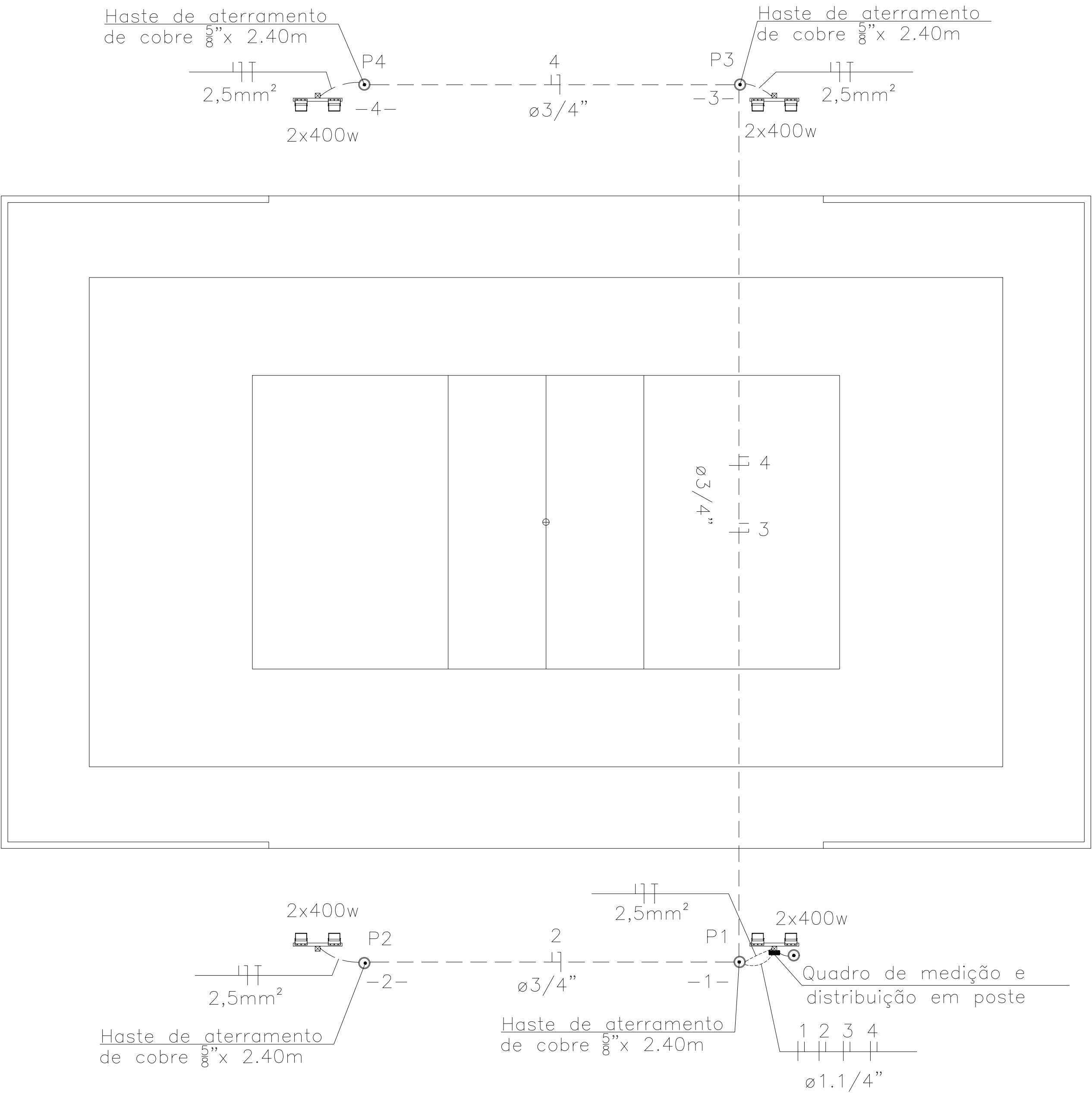
01 PLANTA BAIXA esc.: 1/100
