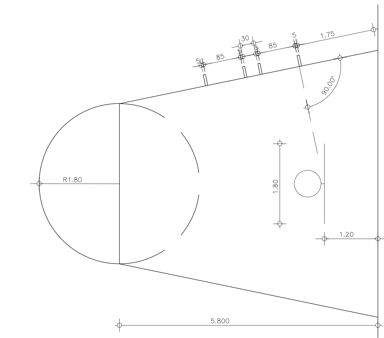
05 ÁREA RESTRITIVA DE LANÇE LIVRE P/ BASQUETE esc.: 1/50
