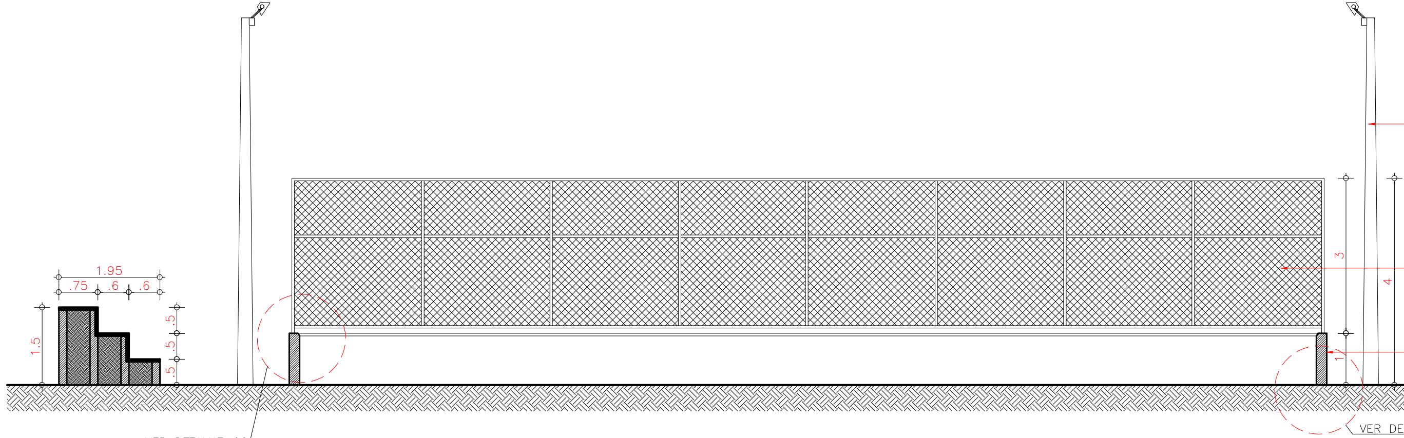
03 CORTE BB" esc.: 1/75
