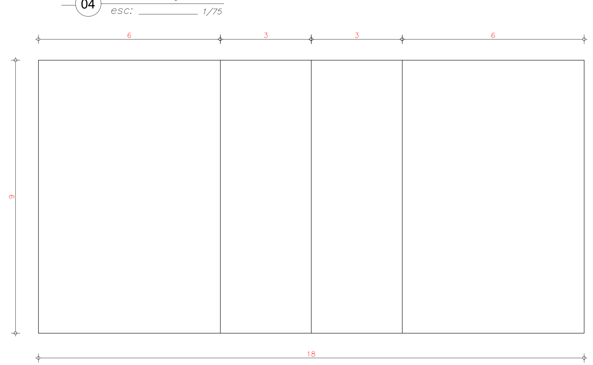
06 DEMARCAÇÃO - VOLEIBOL esc.: 1/75
