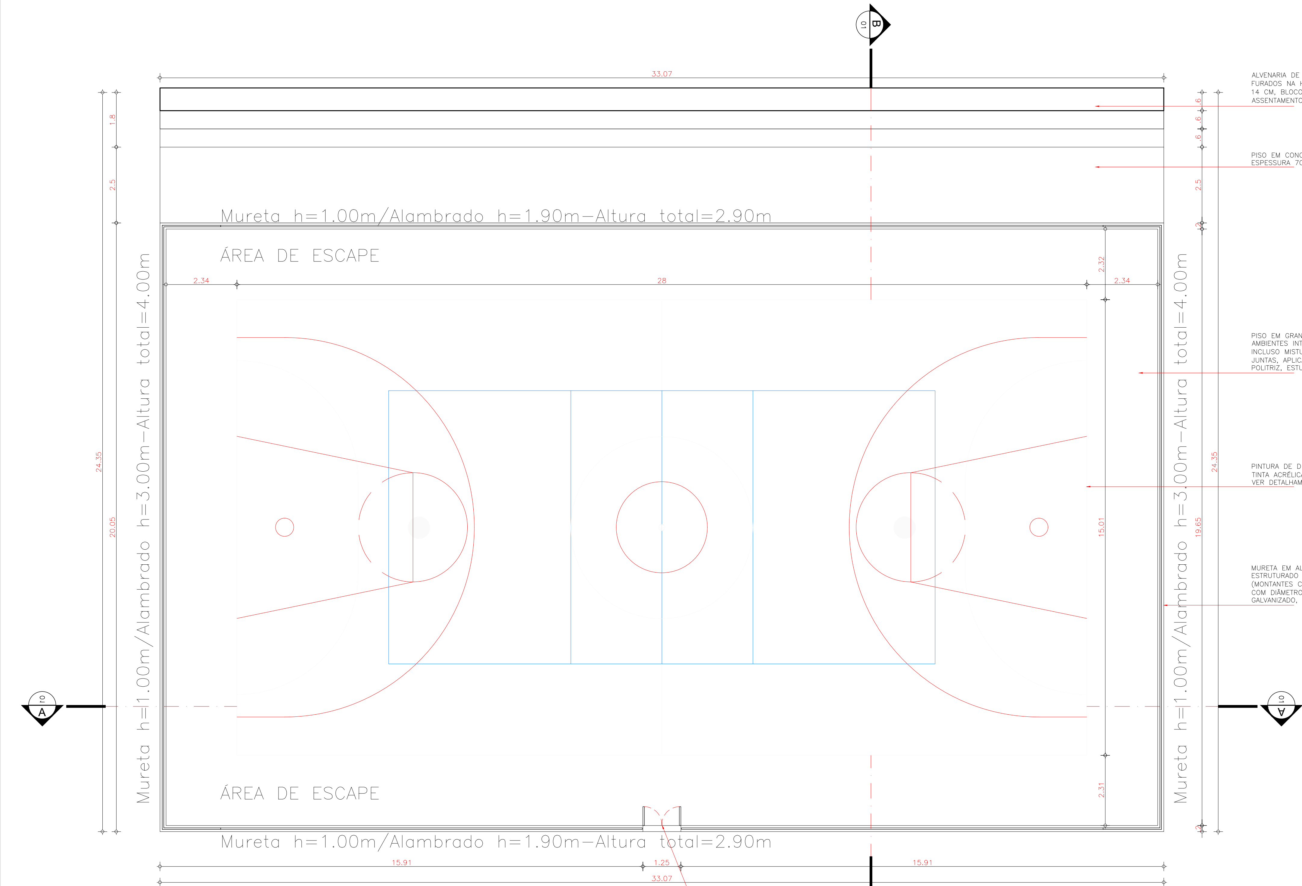
01 PLANTA BAIXA esc.: 1/75
