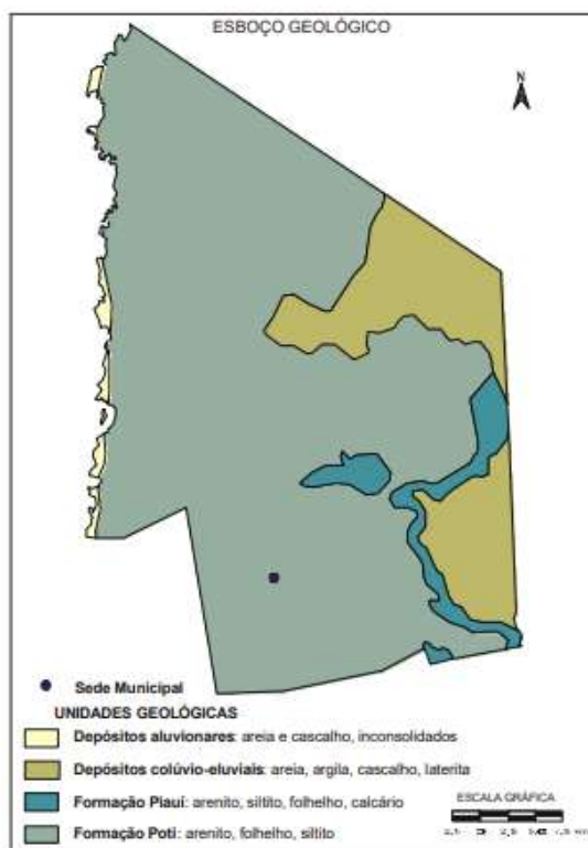
Figura 3 - Esboço geológico do município.
