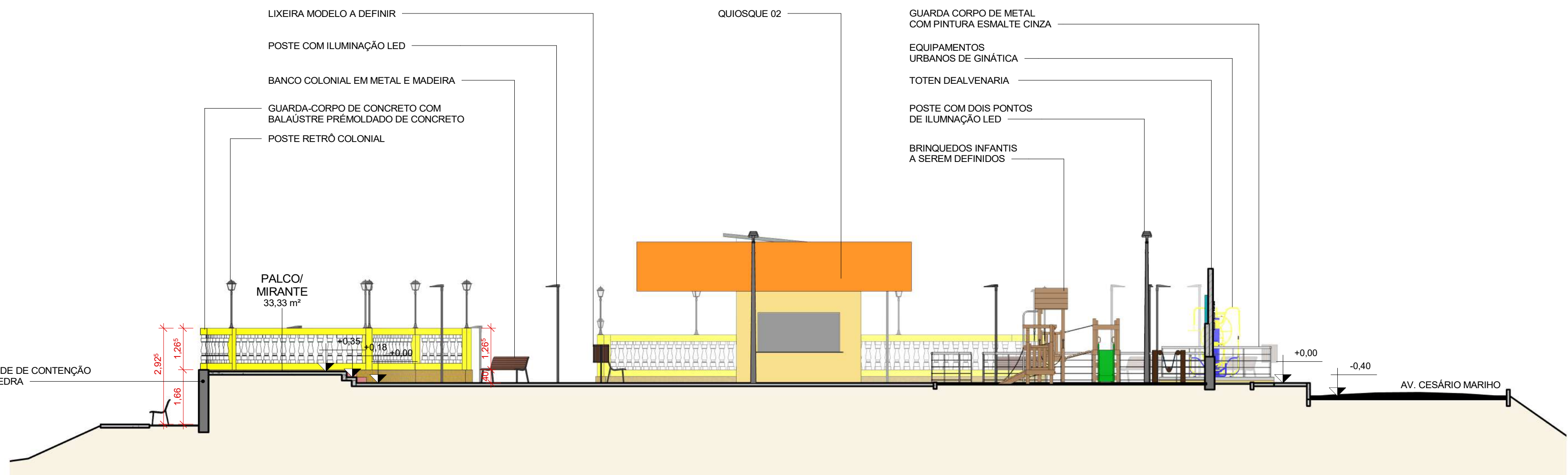
2 CORTE A ESCALA 1:100
