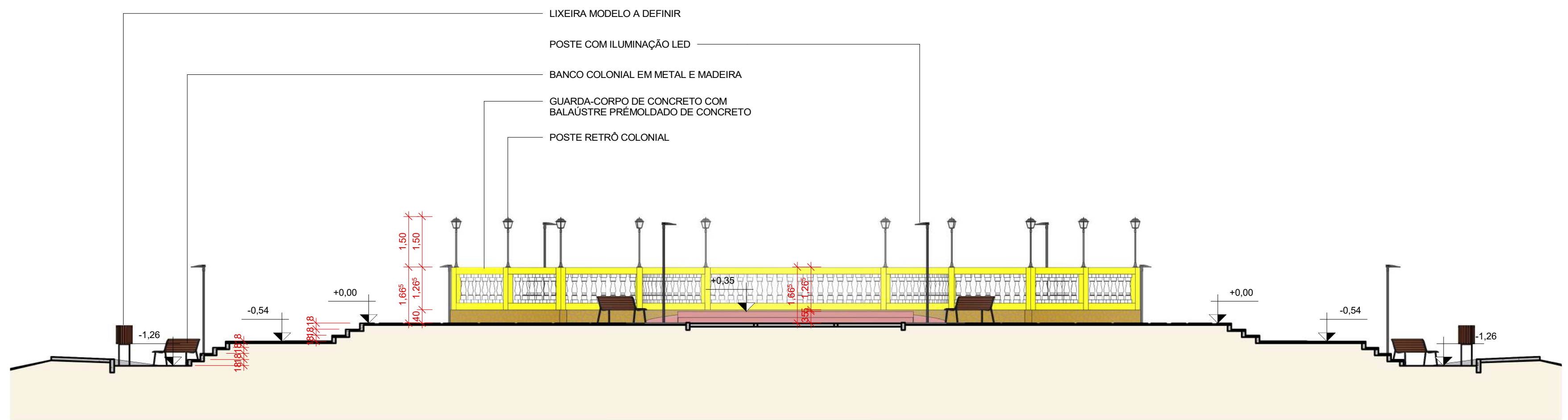
3 CORTE B ESCALA 1:100
