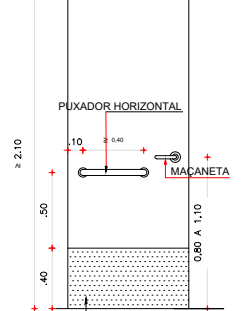
ELEVACÃO FRONTAL ESCALA 1:50
