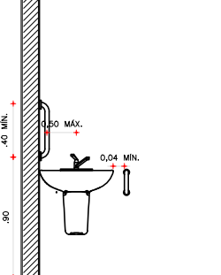
ELEVACÃO FRONTAL ESCALA 1:50
