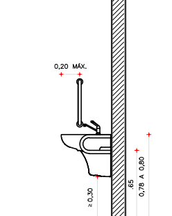
ELEVACÃO LATERAL ESCALA 1:50
