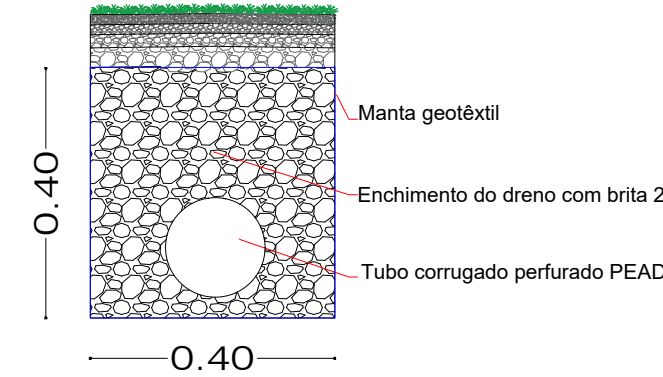
DETALHE 2 - DRENO Sem escala
