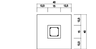
BLOCOS E PILARES ESCALA: 1/25
