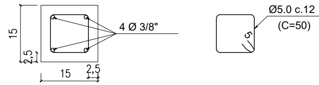
DETALHE FERRAGENS (15x15) ESCALA: 1/10
