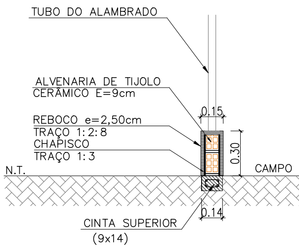
DETALHE DAS FUNDAÇÕES DA MURETA ESCALA: 1/25
