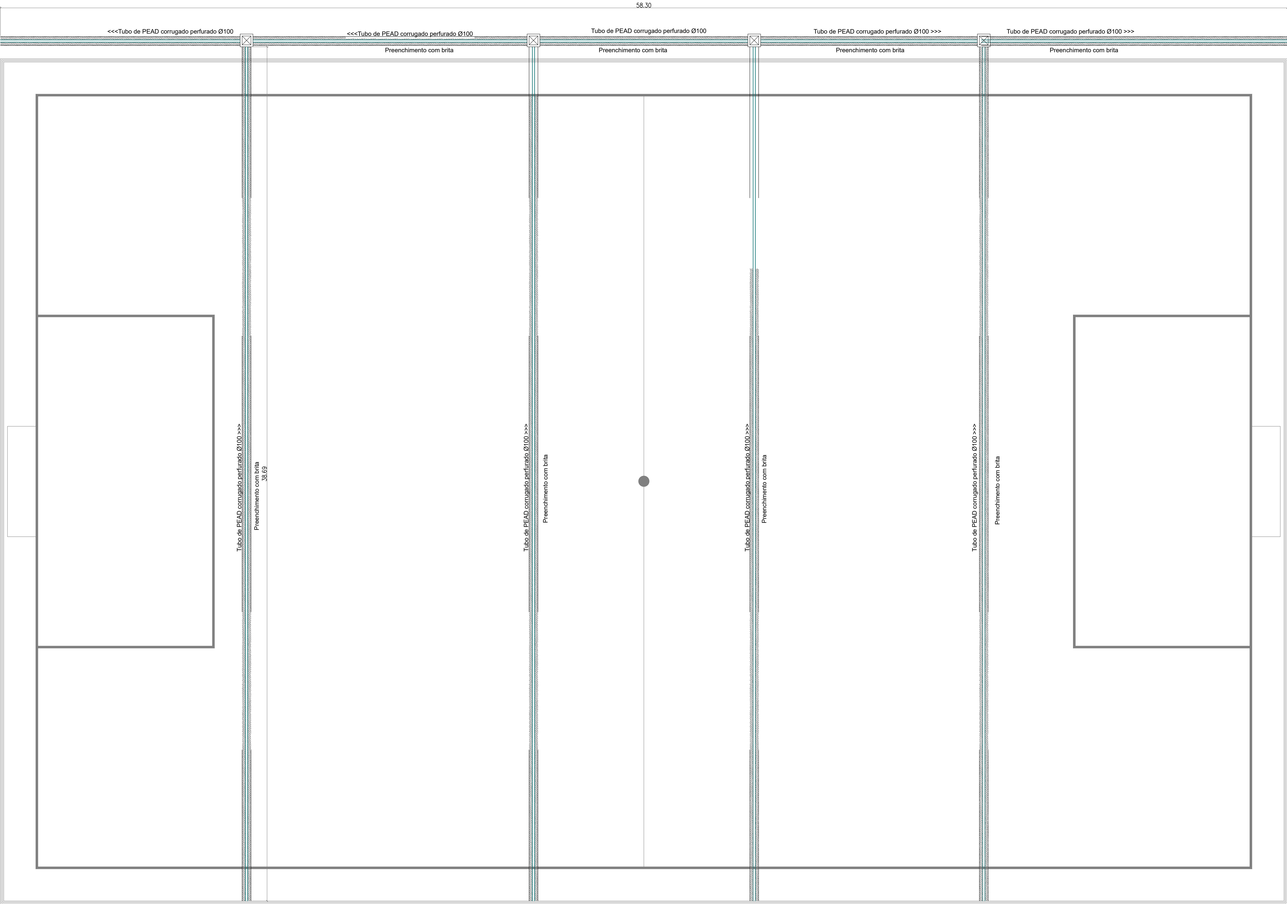
DRENAGEM ESCALA: 1/100
