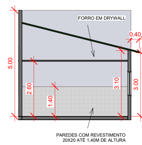
5 Corte BB 1 : 100
