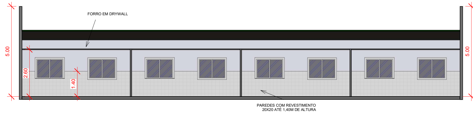
4 Corte AA 1 : 100
