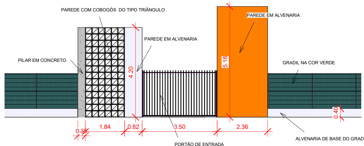
6 Detalhe Alvenarias Fachada 1 : 100
