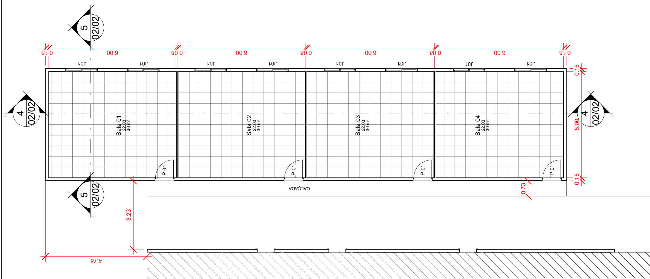
1 Salas de Aula 1 : 100
