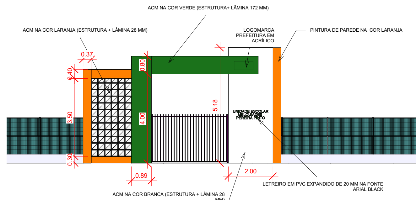
7 Fachada 1 : 100
