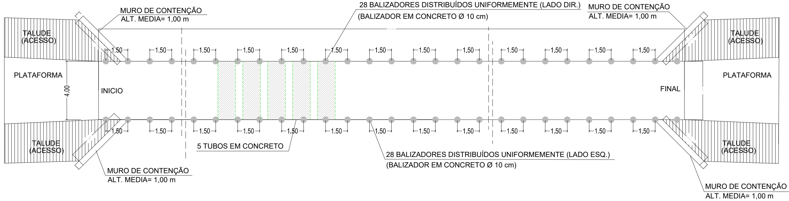
PLANTA BAIXA - PASSAGEM MOLHADA ESCALA 1/150
