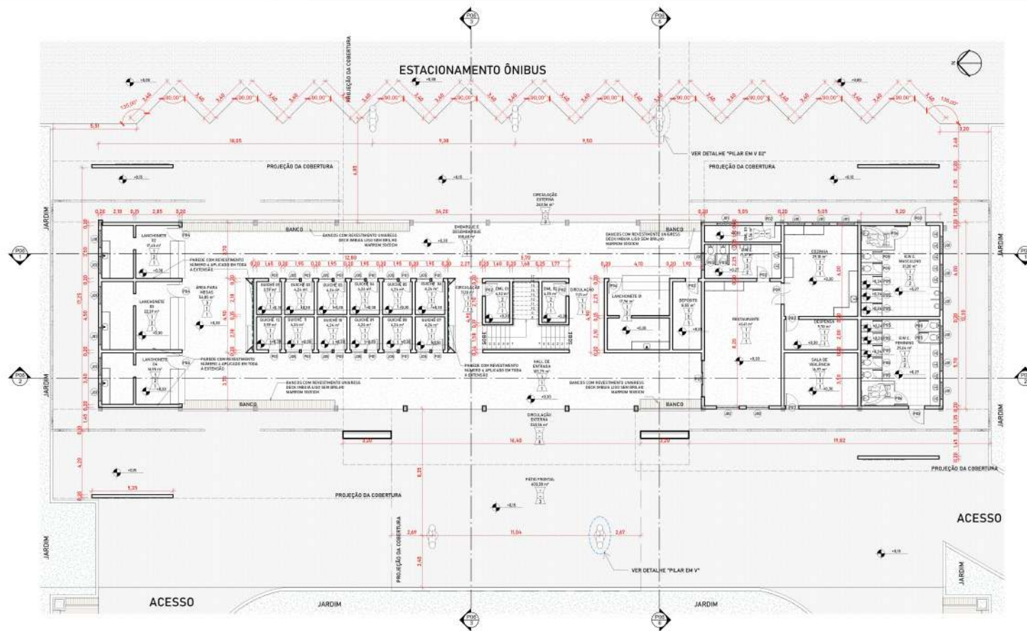
1 TÉRREO ESCALA 1:120
