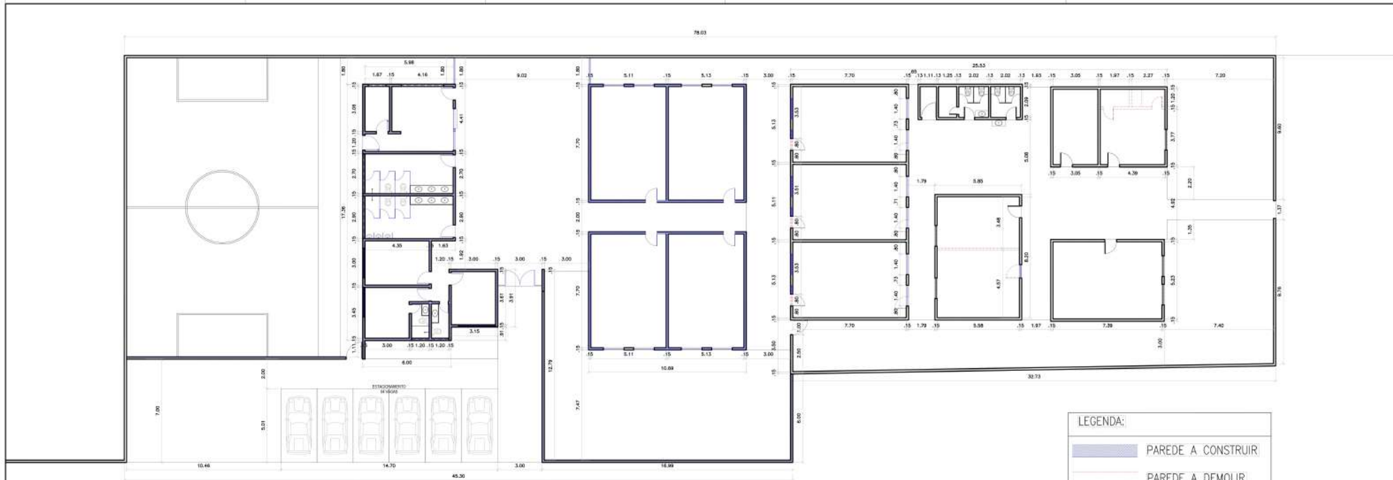
PLANTA BAIXA REFORMA ESC. 1/125
