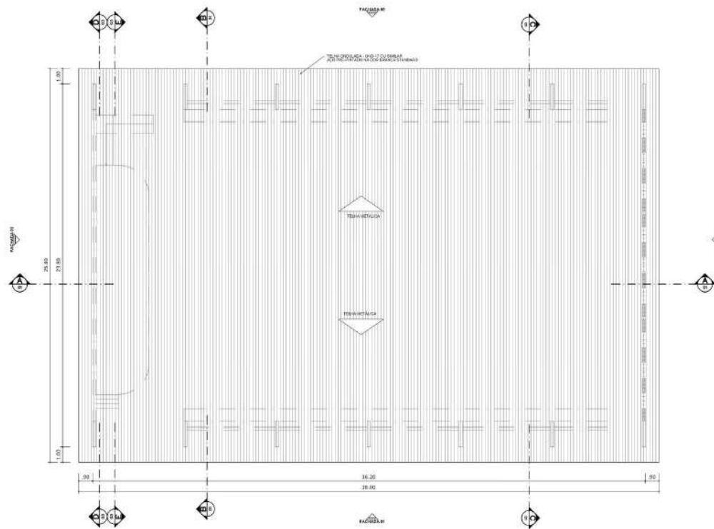
PLANTA DE COBERTURA ESCALA 1:125
